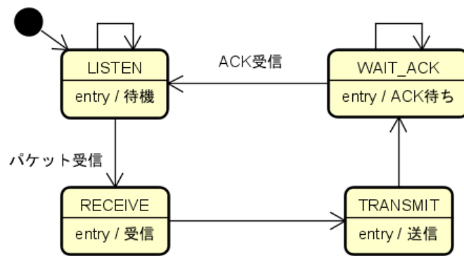
図 3.4: 状態遷移図の例
