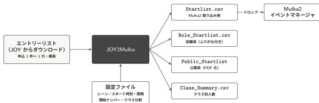
図 14 エントリーから Mulka2 までのデータの流れ
