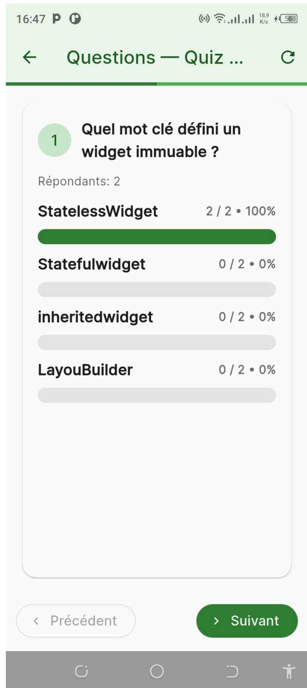
FIGURE 3.14 : Résultats d'une question de quiz Synthèse : nombre de répondants, barres de pourcentage par option, navigation entre les questions. Statistiques calculées en temps réel depuis Supabase.
