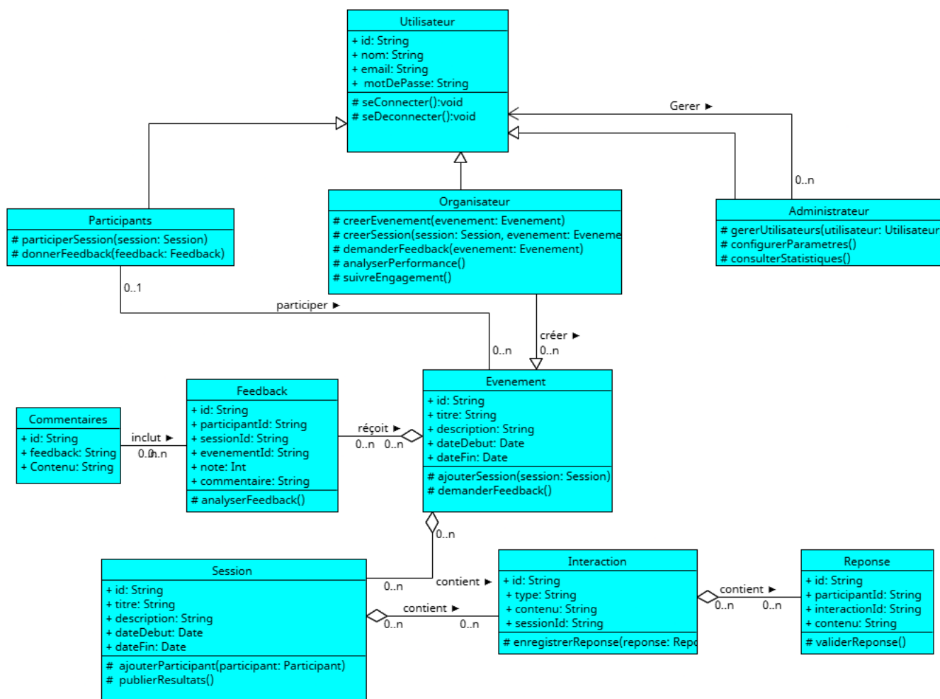
FIGURE 2.5 : Diagramme des classes
