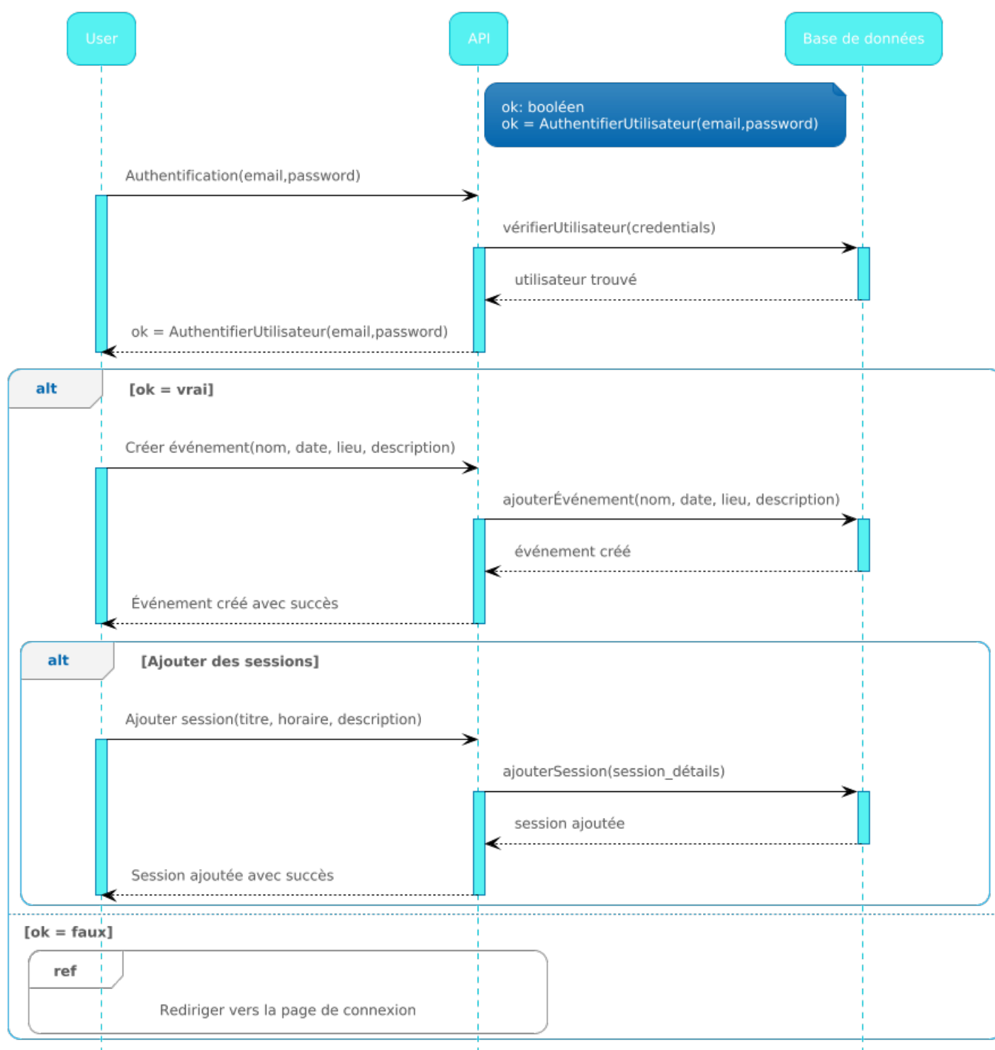
Figure 2.17: Diagramme de séquence pour la création d'un événement
