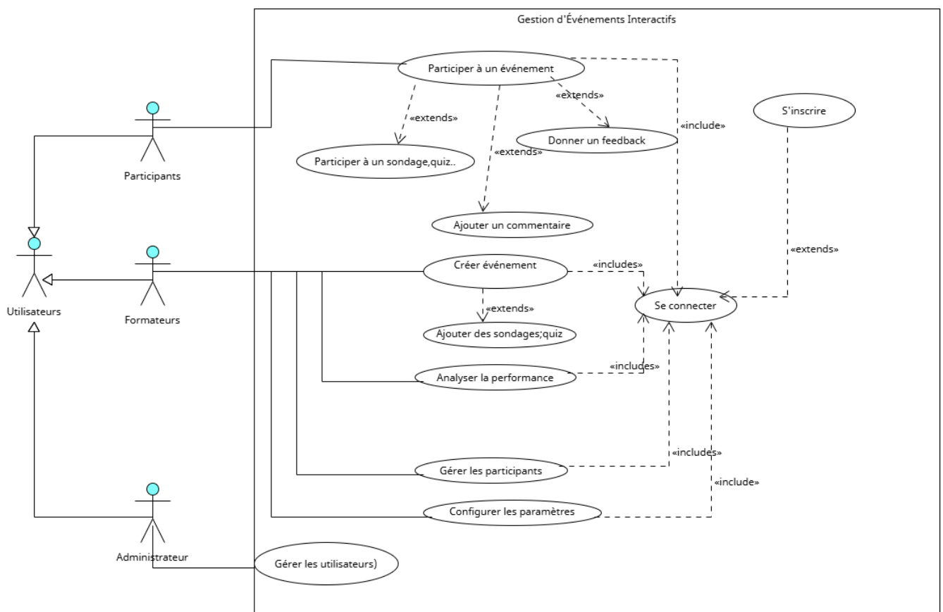
Figure 2.13: Diagramme de cas d'utilisation
