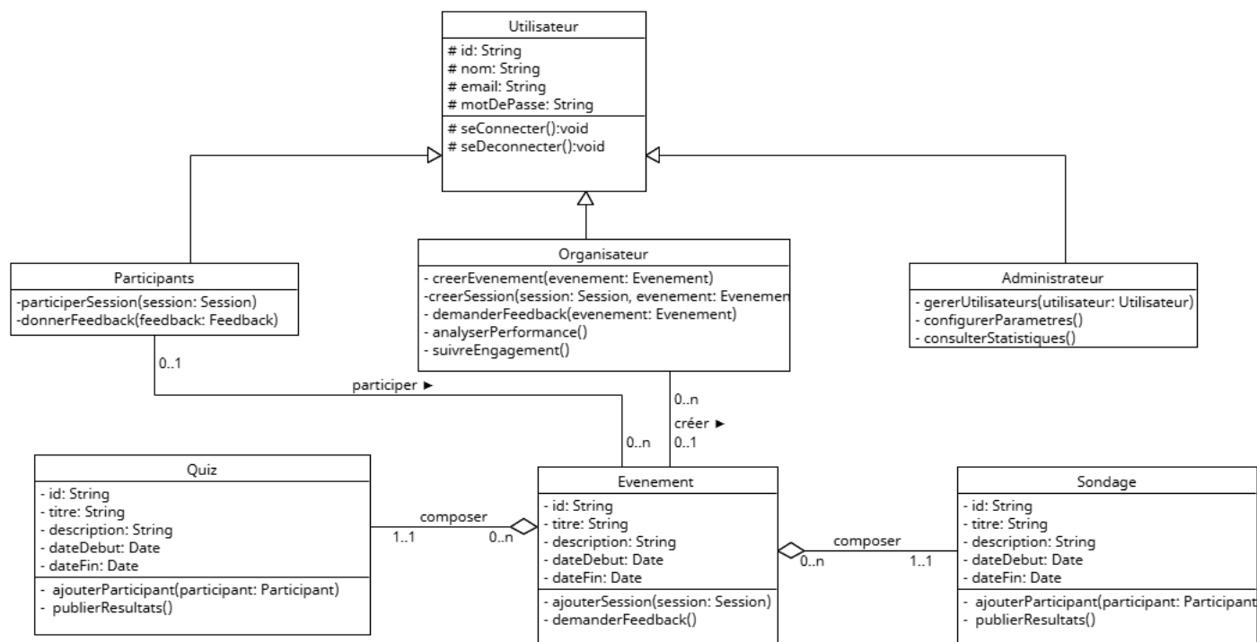
Figure 2.14: Diagramme des classes
