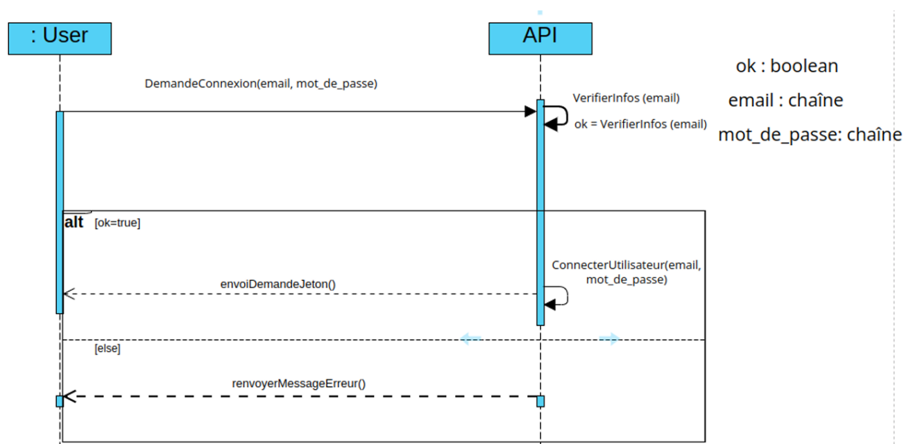
Figure 2.16: Diagramme de séquence pour la connexion
