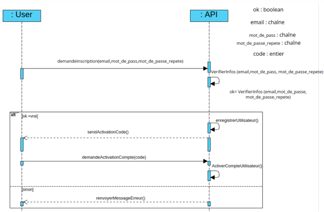
Figure 2.15: Diagramme de séquence pour l'inscription
