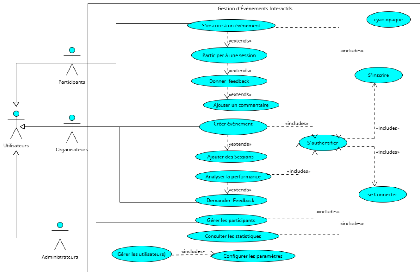
FIGURE 3.4 : Diagramme de cas d'utilisation
