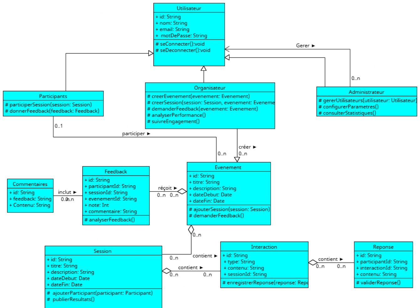
FIGURE 3.5 : Diagramme des classes
