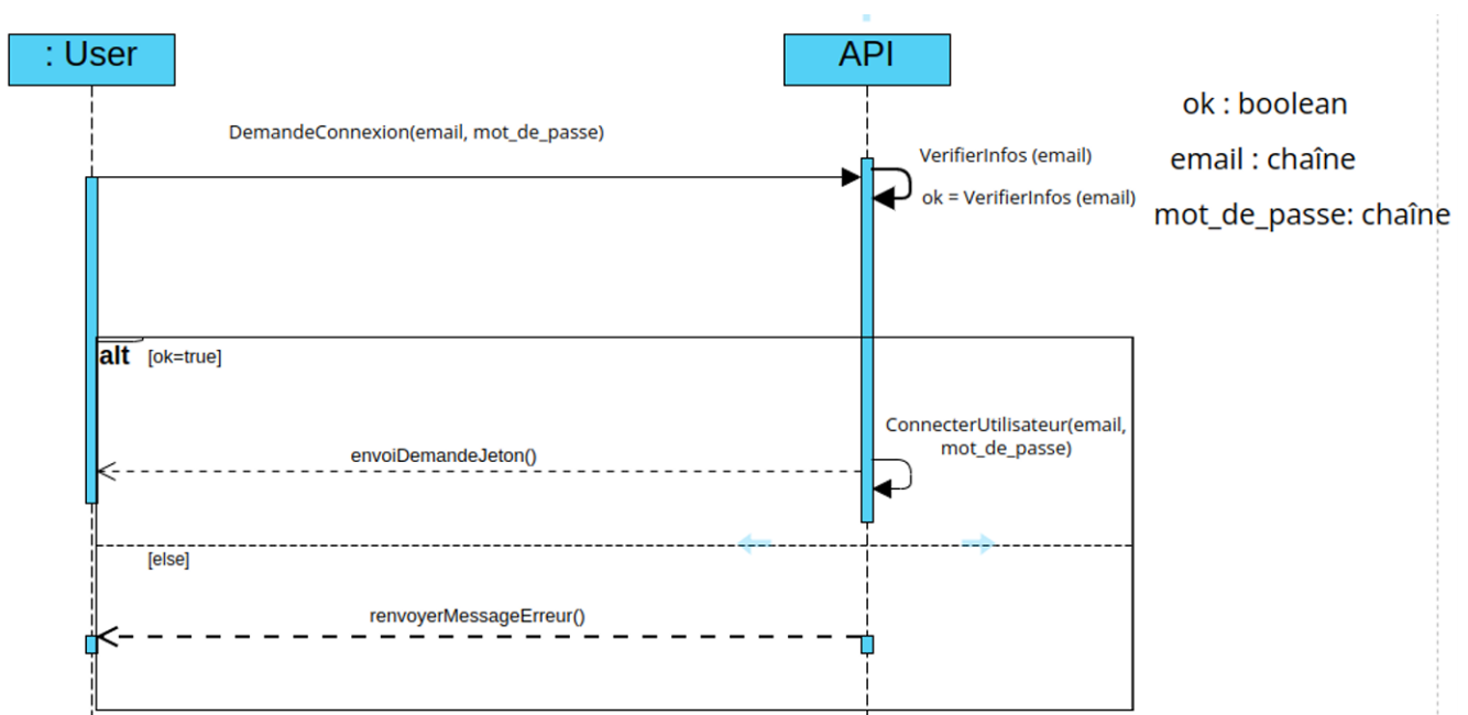
FIGURE 3.7 : Diagramme de séquence pour la connexion
