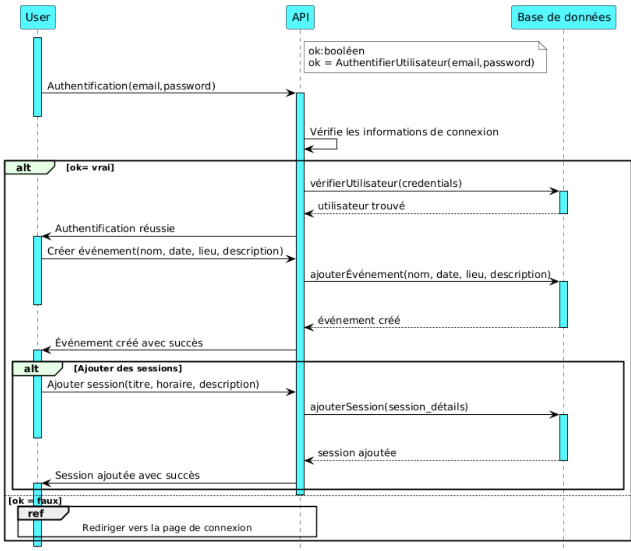
FIGURE 3.8 : Diagramme de séquence pour la création d'un événement
