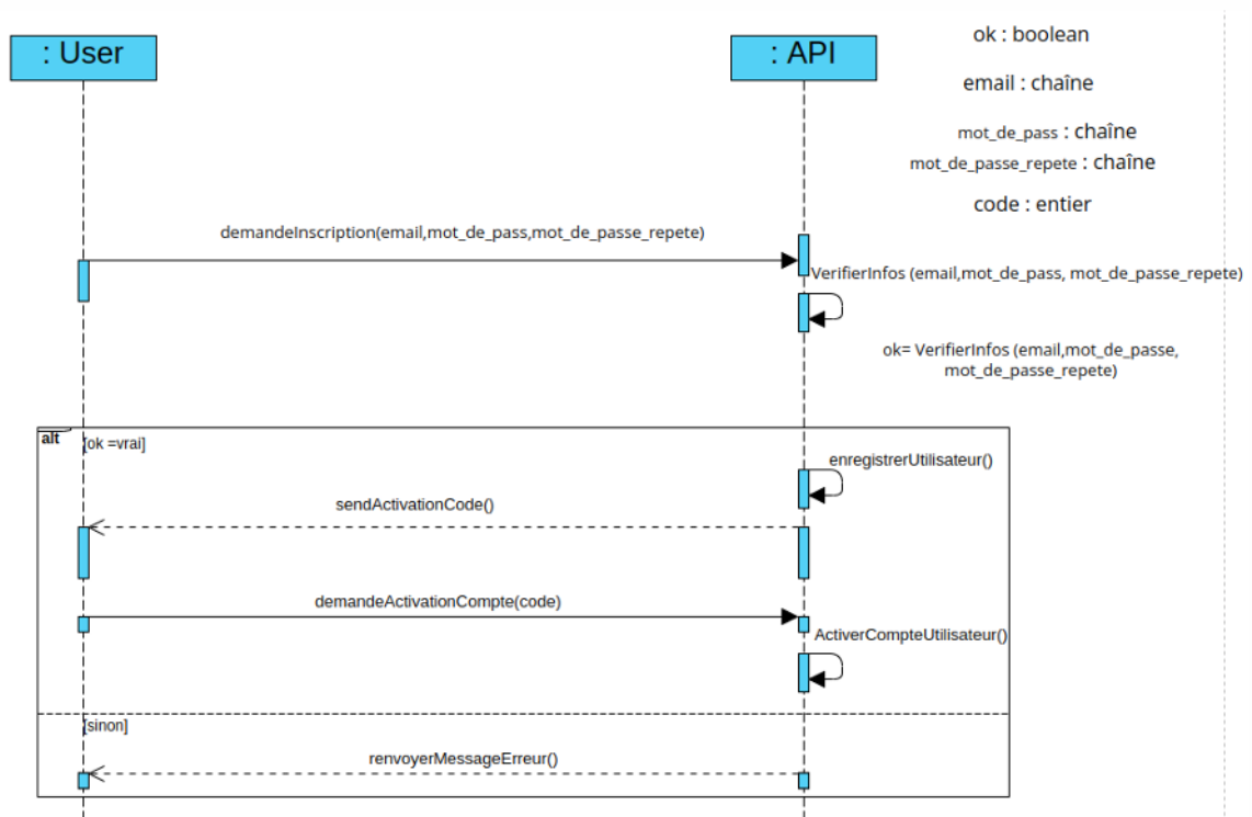
FIGURE 3.6 : Diagramme de séquence pour l'inscription
