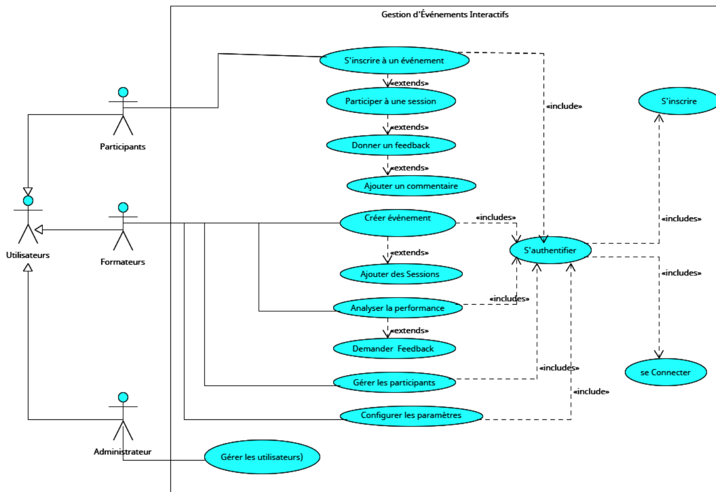
FIGURE 2.4 : Diagramme de cas d'utilisation
