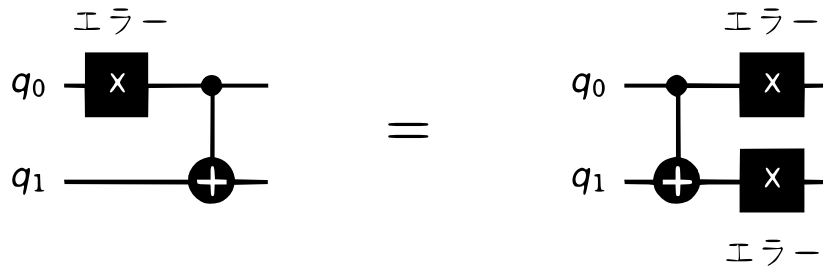
Figure 22: エラー伝播の模式図
