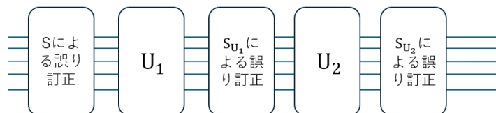
Figure 19: エラー訂正回路
