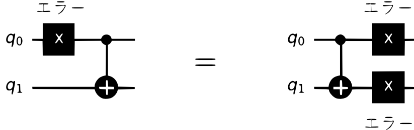
Figure 22: エラー伝搬の模式図
