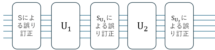
Figure 19: エラー訂正回路
