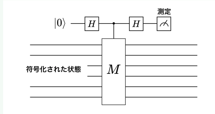
Figure 18: 一般のシンδροーム測定回路
