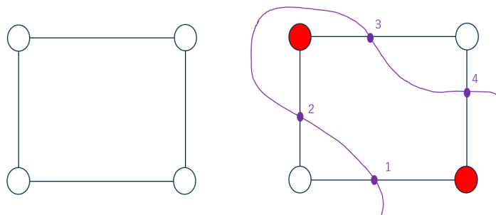
Figure 15: 正方形のグラフ（左側）、およびその max-cut(右側)
