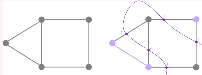
Figure 14: max-cut 問題の模式図。左図が与えられたグラフで、右図が紫と白に頂点をグループ分けした図
