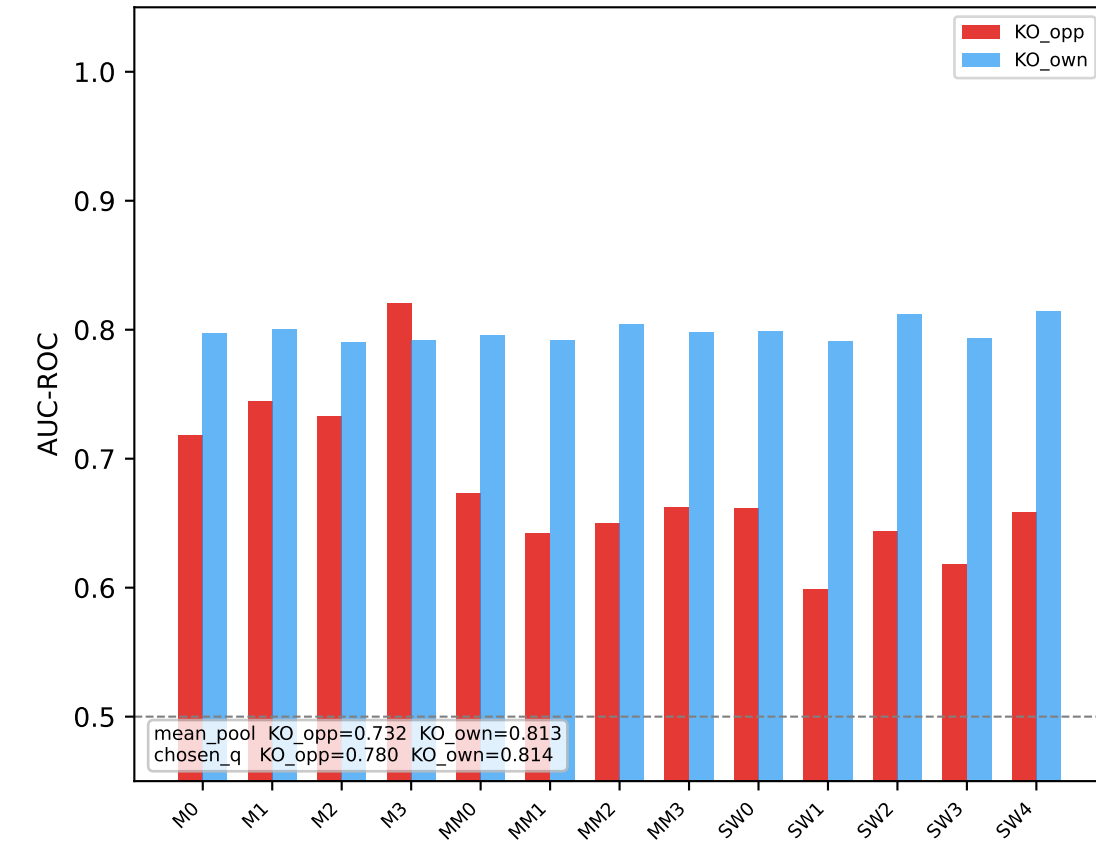
Probe 4 — KO next turn AUC
