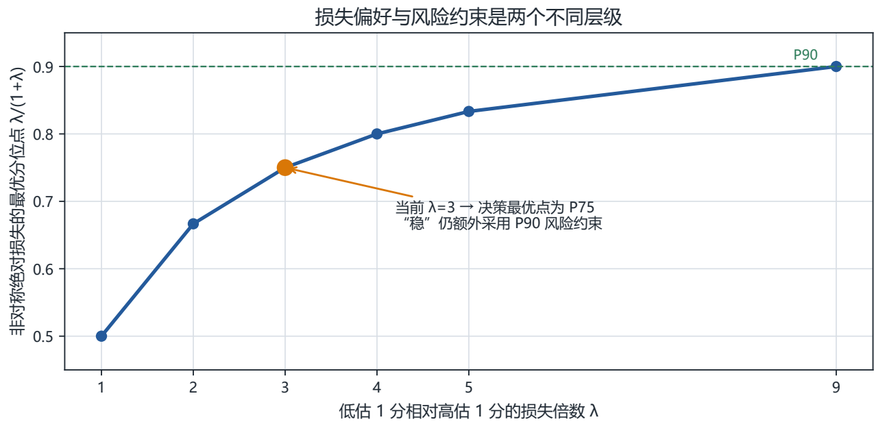
图 19 非对称损失倍数与最优分位点的关系。若要仅靠损失函数得到 P90，低估损失需设为高估的 9 倍；当前 \lambda = 3 对应 P75。 曲线由式 (21) 直接计算。
