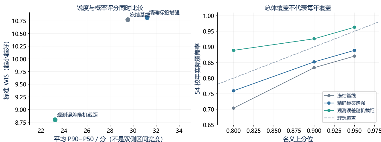
图 29 左图同时衡量上尾锐度和标准概率评分，右图比较三个上分位的总体覆盖。覆盖接近对角线仍不能保证新年份、事件学校或低证据学校的条件覆盖。
