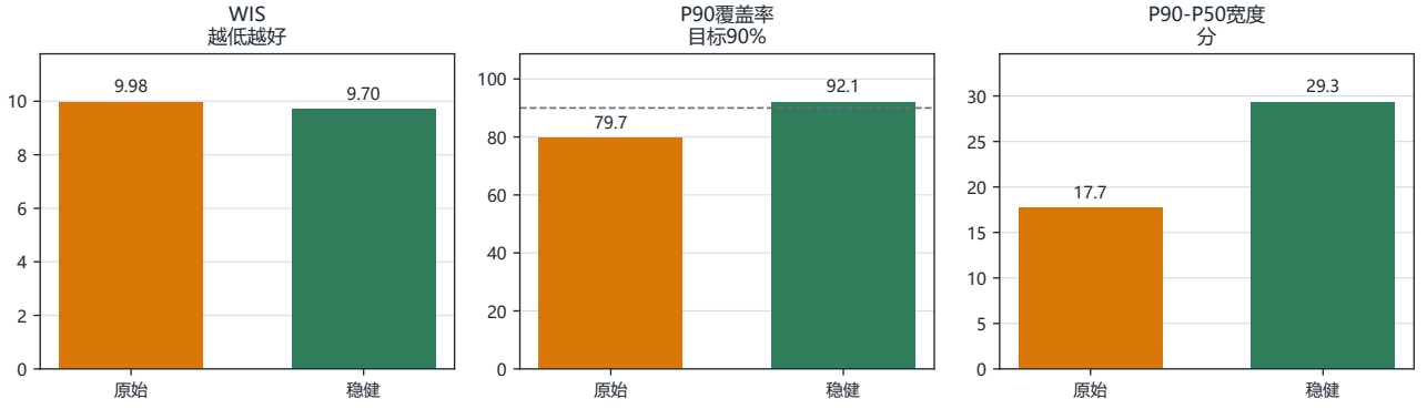
图 17 严格嵌套校准的三维权衡。稳健上界同时改善 P90 覆盖距离与 WIS，但以更宽区间为代价；因此评价不能只看覆盖率。
