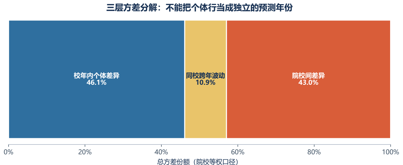
图 10 院校等权的三层方差分解。校年内个体差异与院校间差异均占较大份额，因此既不能只研究全国混合分布，也不能把同一校年的个人记录当作时间外样本扩容。
