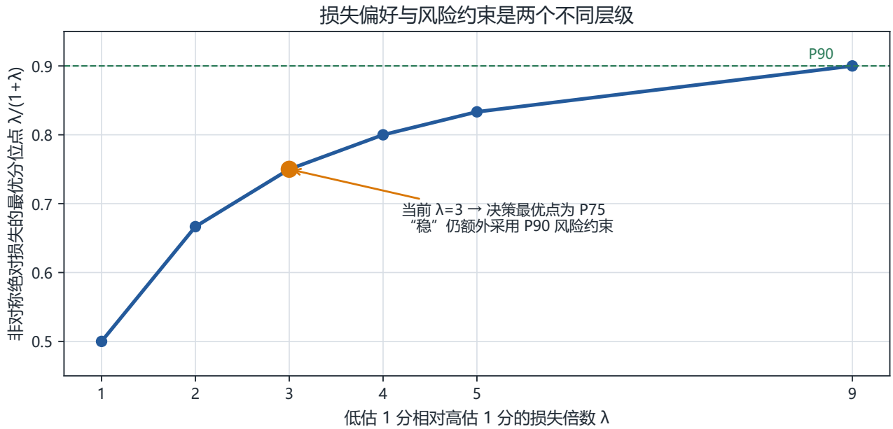
图 19 非对称损失倍数与最优分位点的关系。若要仅靠损失函数得到 P90，低估损失需设为高估的 9 倍；当前 \lambda = 3 对应 P75。 曲线由式（35）直接计算。
