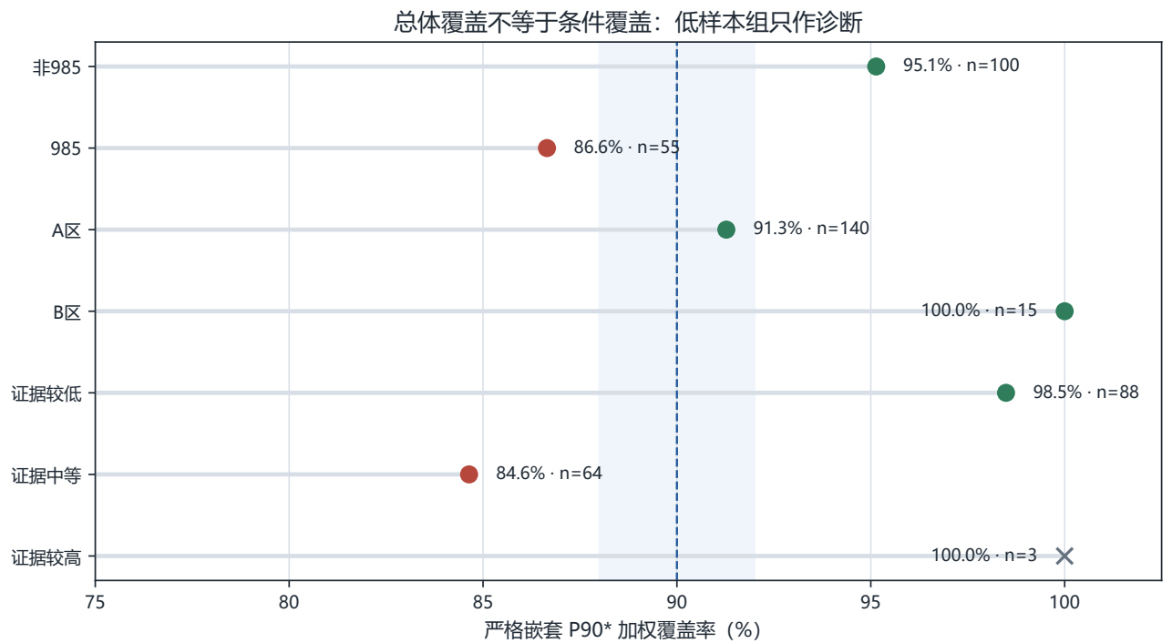
图 34 严格嵌套 P90* 的条件覆盖诊断。点位显示加权覆盖率，文字同时给出原始记录数；叉号表示样本少于 10 条，只可作为风险提示。图形把“总体达标但 985 子组偏低”直接呈现出来，避免用总体 92.1% 掩盖分组失配。
