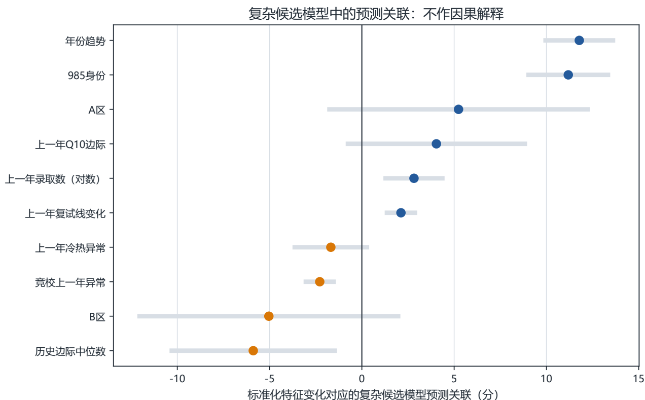
图 23 复杂候选模型的主要预测关联及后验标准差。横轴为标准化输入变化对应的模型关联，误差线反映参数不确定性；静态类别和小样本系数存在较宽区间。
