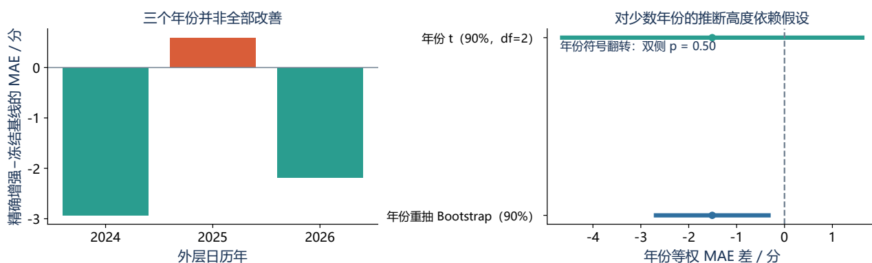
图 35 年份层面的样本数而非考生人数约束泛化推断。不同假设导致不同区间；图中负值仅表示当前样本的增强误差较小。
