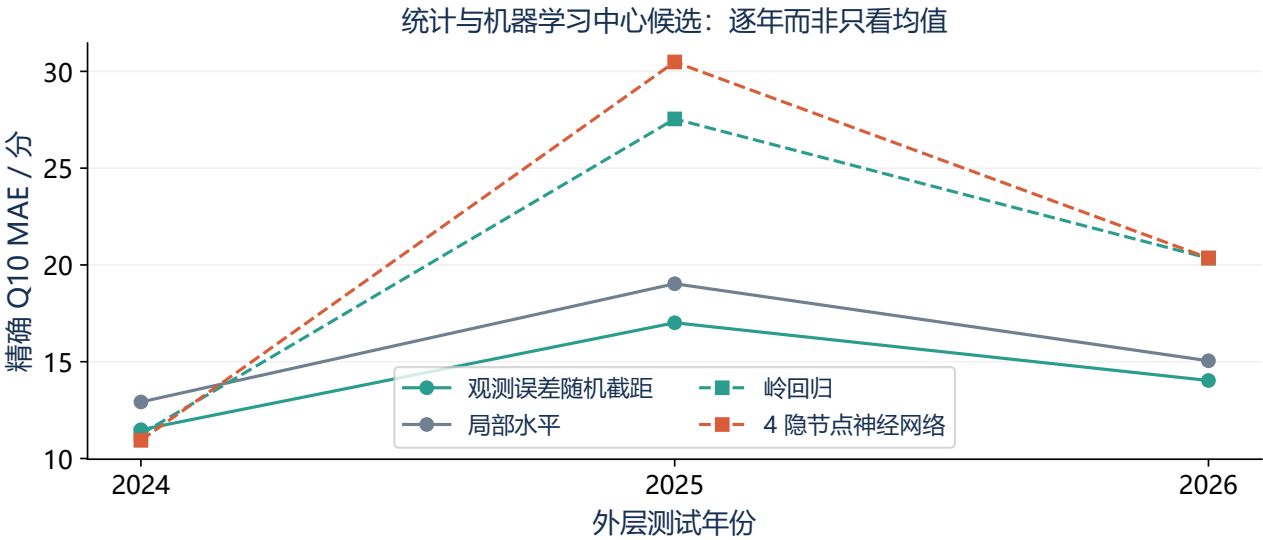
图 30 同一批测试校年、同一中心目标下的逐年误差。网络在 2024 年误差较低，却在 2025 年明显恶化；单个好看的年份不足以支持跨年稳定泛化。
