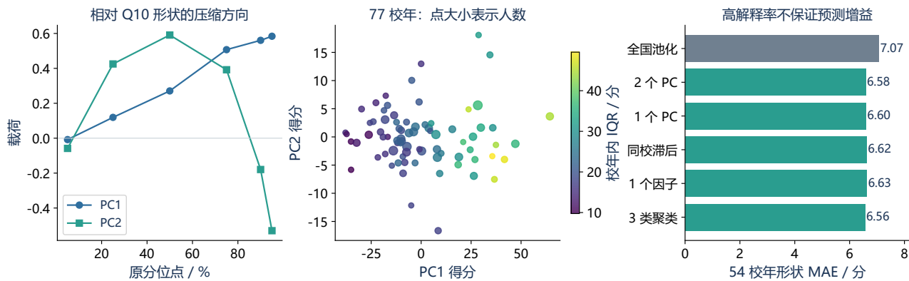
图 31 载荷解释压缩了哪类分位差异；得分图的颜色表示 IQR、点大小表示名单人数；右图用真正下一年形状误差检验“可压缩”是否转化为“更可预测”。全样本坐标只用于描述，各预测原点另拟合训练期基底。
