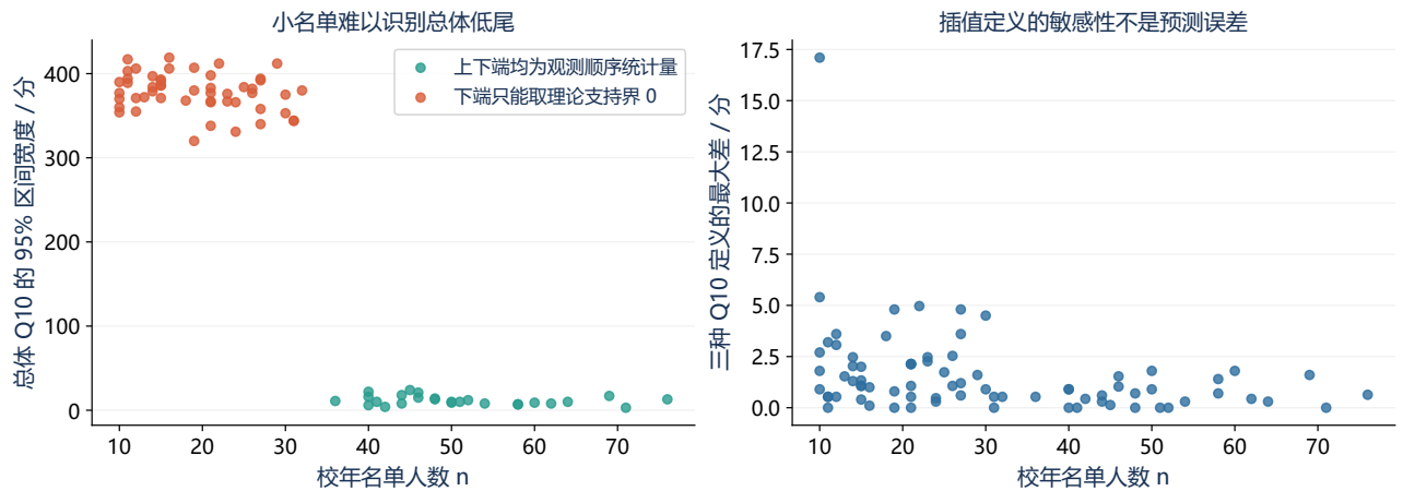
图 27 名单规模影响潜在总体低尾的可识别性，也影响不同经验分位定义的差异；两个纵轴都不等于未来 Q10 的预测误差。来源：审计名单的校年聚合与二项顺序统计计算。
