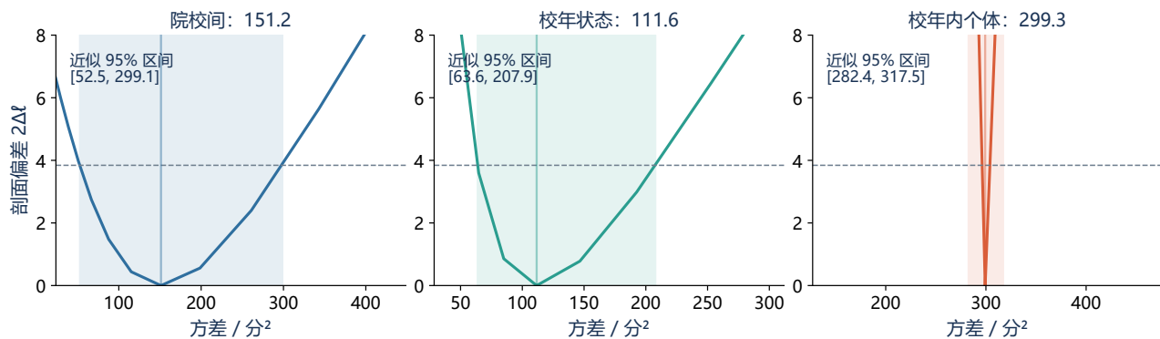
图 28 剖面曲线横轴为方差，阴影为近似 95% 区间，虚线为卡方工作阈值。校年内个体方差的信息量明显大于跨校、跨年的方差信息量。
