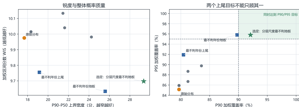
图 33 九种校准候选的多目标比较。左图同时检查锐度与 WIS，右图检查 P90 和 P95 是否共同达到名义目标；仅提高一个覆盖率并不足以上线。选定方案不是每个单指标的冠军，而是在当前冻结规则下同时越过两个上尾目标，代价是更宽区间。由于候选仍复用 2025–2026 两个外层年份，本图用于解释选择，不构成独立验证。
