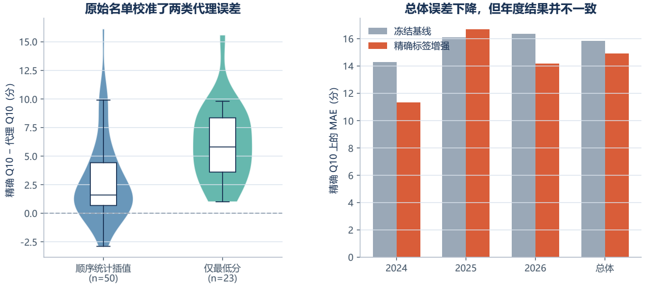
图 3 逐人原始分数对代理误差与中心预测的双重检验。左图显示顺序统计插值和仅最低分两类代理都存在系统向下偏差，后者更明显；右图在 54 个 2024–2026 年精确回测校年上比较冻结基线与精确标签增强模型。总体 MAE 从 15.83 降至 14.90 分，但 2025 年没有改善，故不能把“总体改善”写成“每年都改善”。
