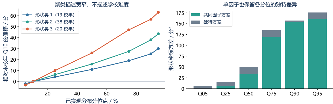
图 32 聚类将 Q10 对齐后的分布分成宽窄不同的形状；因子模型在上分位识别较强的共同展开，同时保留低尾坐标的独特差异。形状类别不是课程派系、院校层级或择校风险等级。
