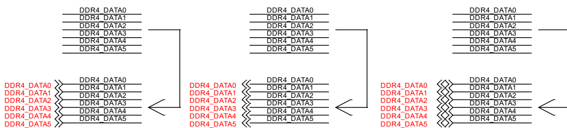
图 2 放置右连接 Off-Page
