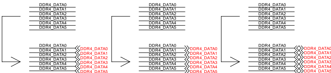
图 3 放置左连接 Off-Page
