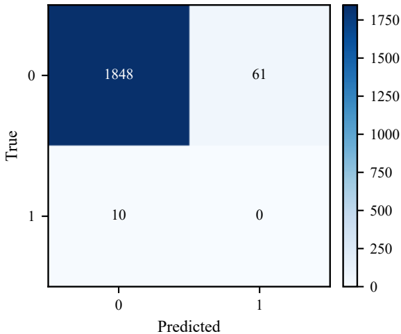
T2 confusion (v1.1.0-INST)
