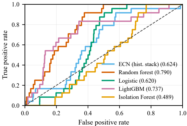
T1 ROC
