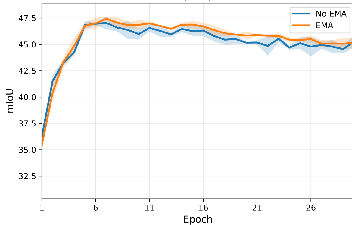
Cityscapes
