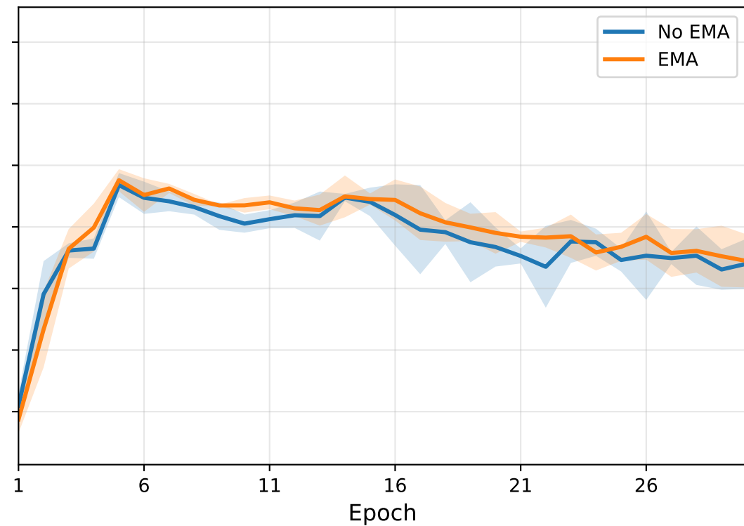
BDD
