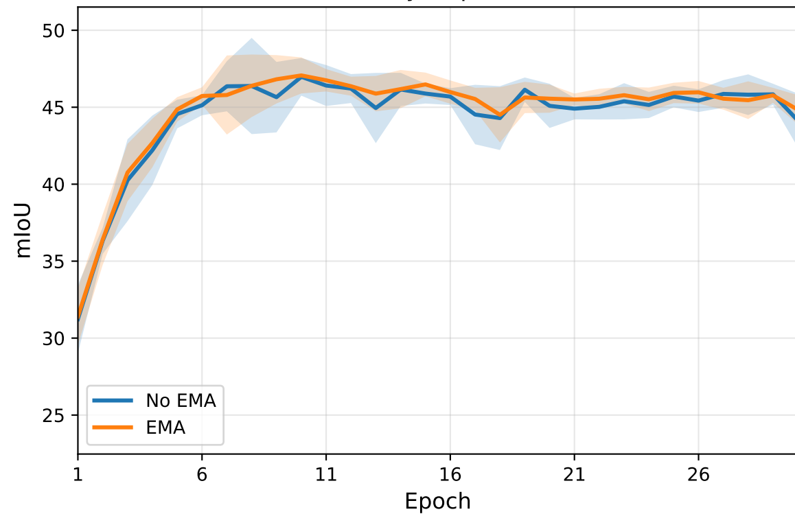
Cityscapes
