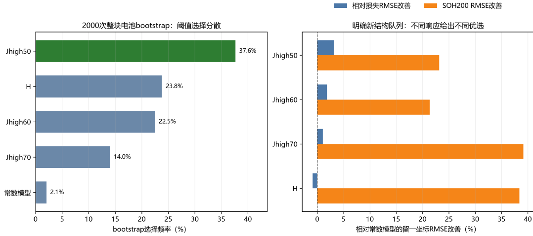
图 6 模型系数稳定性与选择校正
