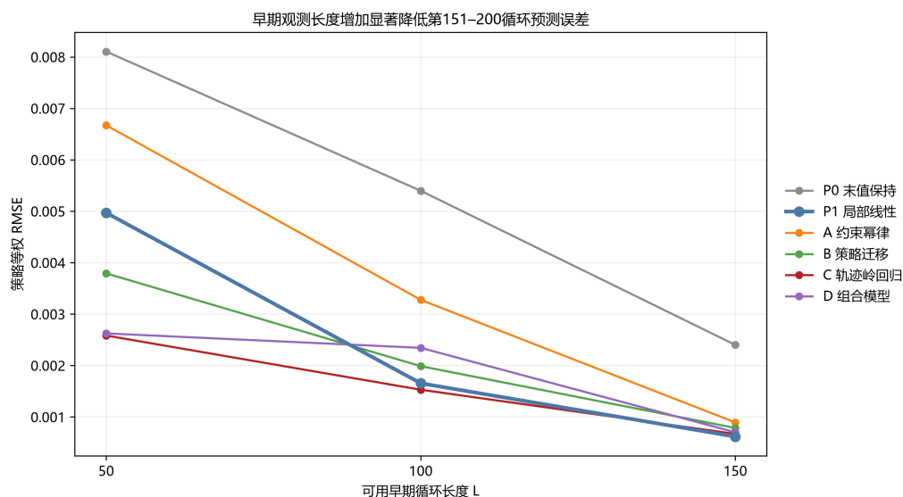
图 7 六候选模型随早期数据长度的 LOBO RMSE
