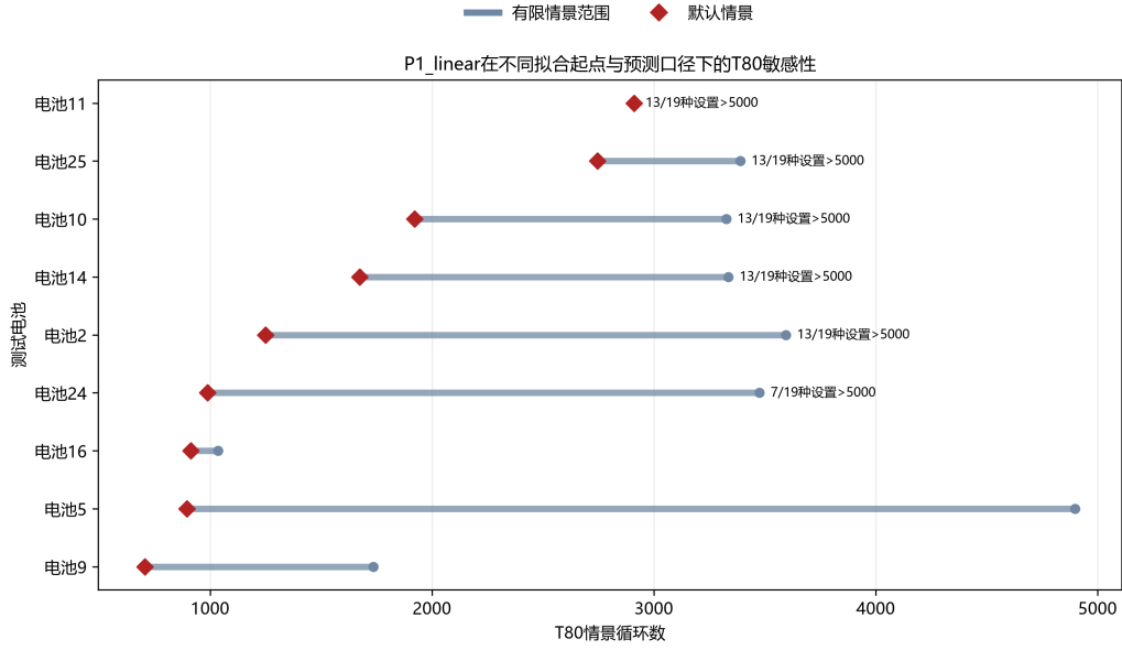
图 9 T_{80} 情景外推敏感性（红菱形为默认情景）
