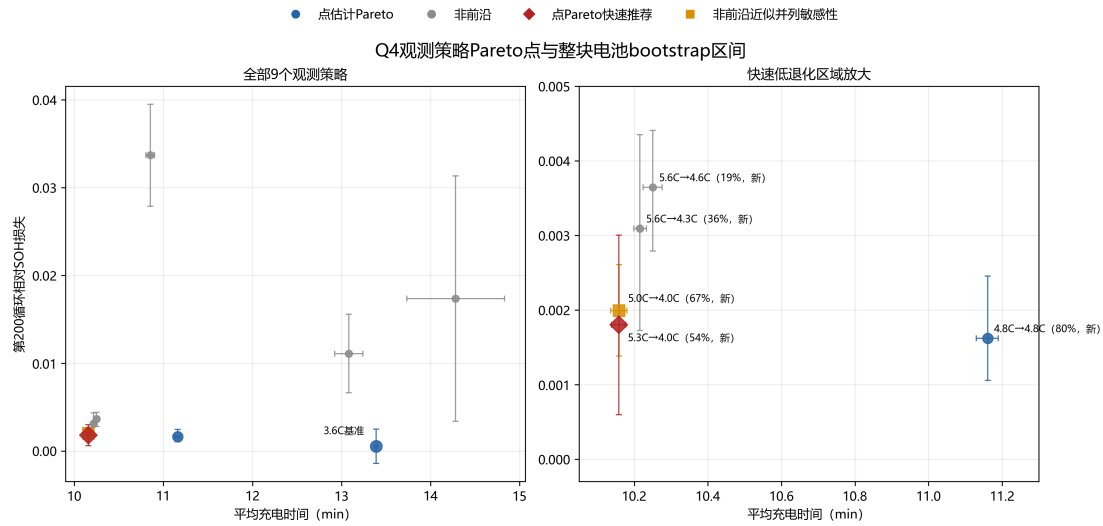
图 10 充电时间-退化 Pareto 前沿与 bootstrap 不确定性
