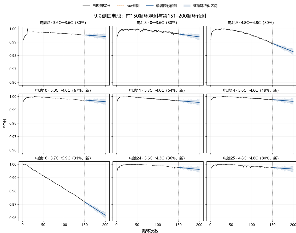
图 8 9 块测试电池 151–200 循环预测（实线单调投影、阴影保守点区间）
