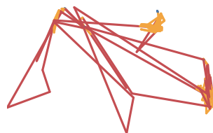
elk-163 Gaussian K=3
