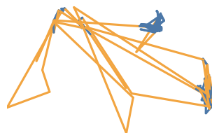
elk-163 Mixture K=2
