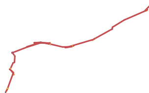
elk-287 Gaussian K=3
