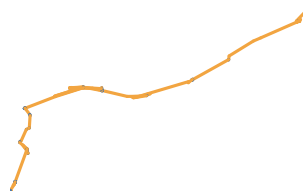
elk-287 Mixture K=2
