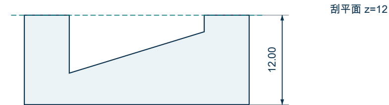
A-A 剖面 / XZ；四腔截面相同
