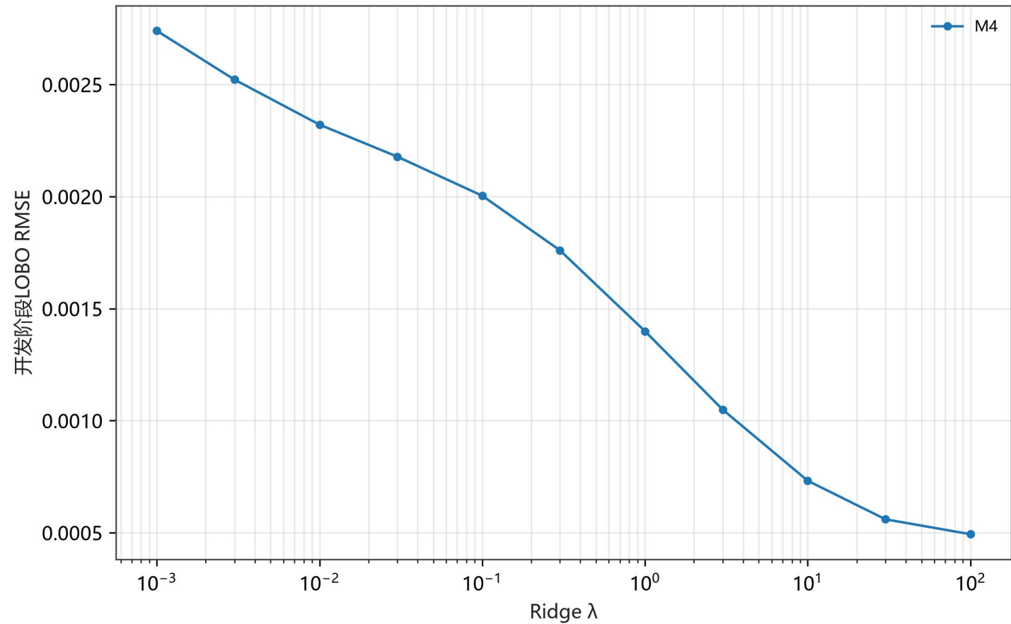
Ridge \lambda 选择诊断 (仅训练电池)
