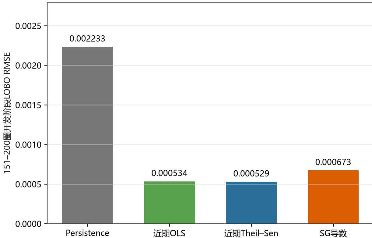
个体趋势Baseline比较 (L=150)
