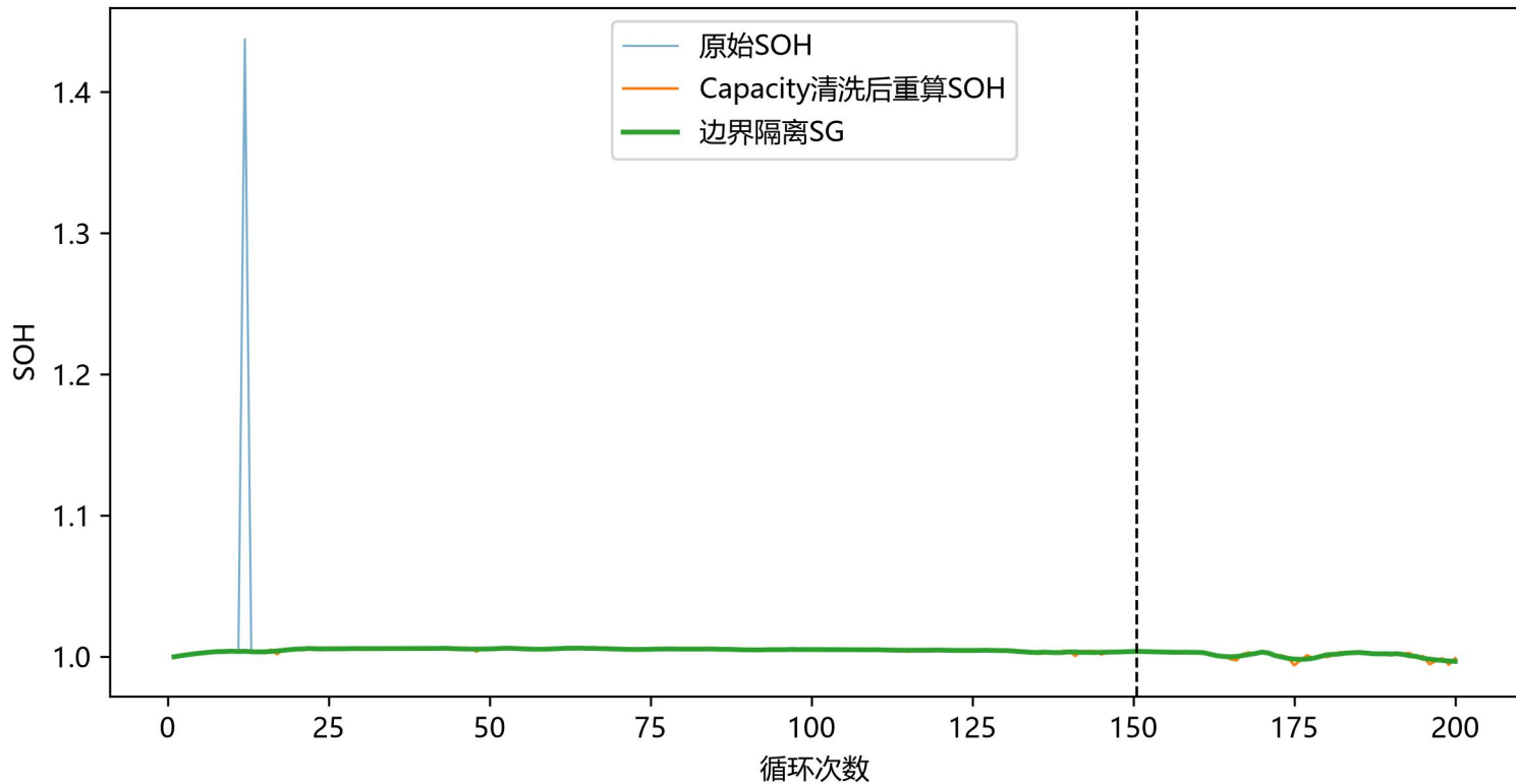
电池1：异常处理与SG平滑
