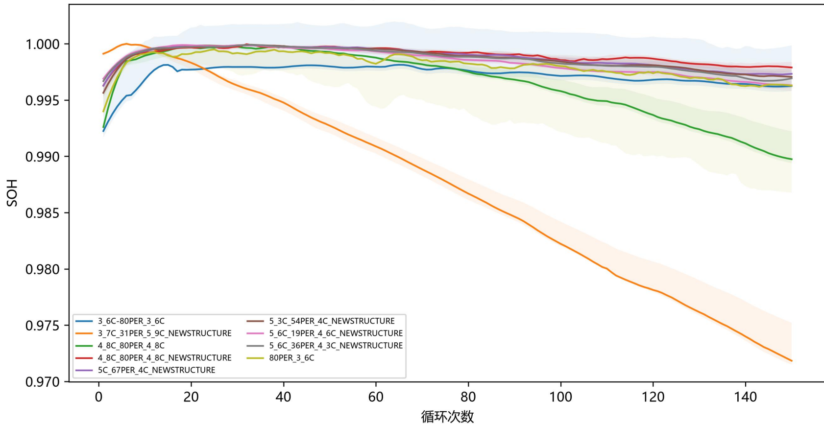
9种策略前150圈SOH中位曲线与IQR
