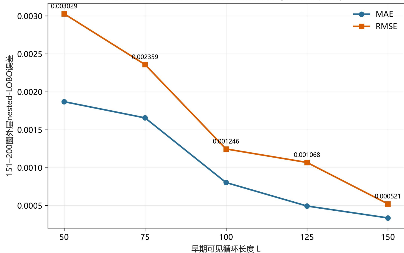
早期数据长度对未来SOH预测精度的影响（无偏外层评价）
