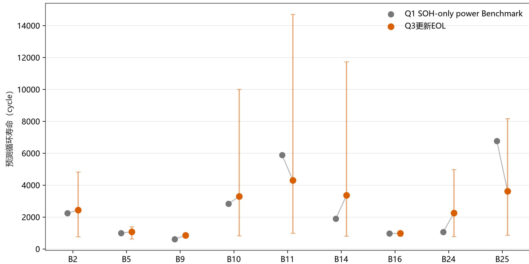
9块测试电池：Q1 Benchmark与Q3预测EOL
