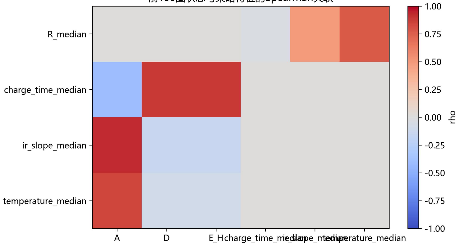
前150圈状态与策略特征的Spearman关联
