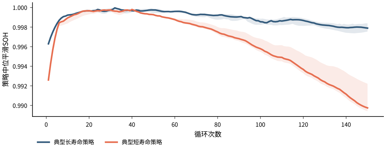
典型长、短寿命策略在早期SOH上已呈现分离
