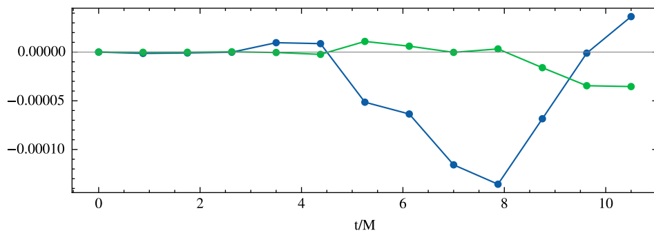
Gamma1
