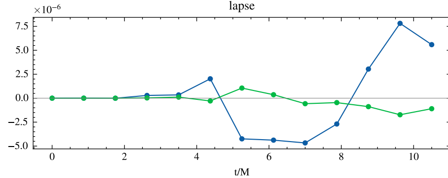
Ex
