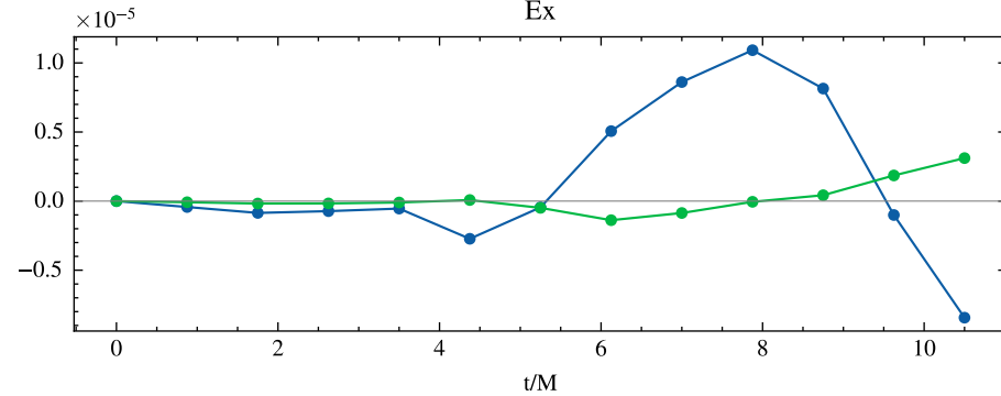
Ex
