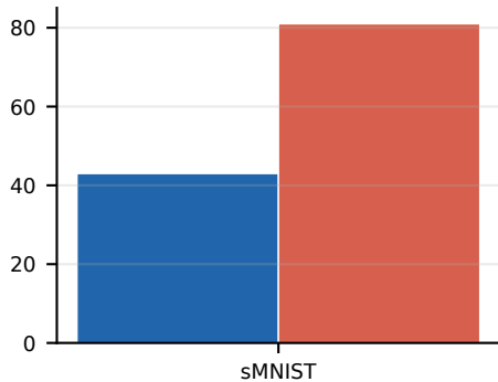
LUD (90% var)
