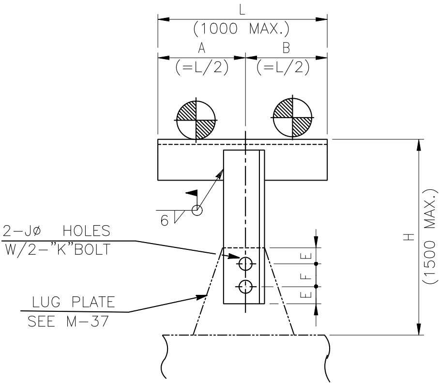
ELEV.
