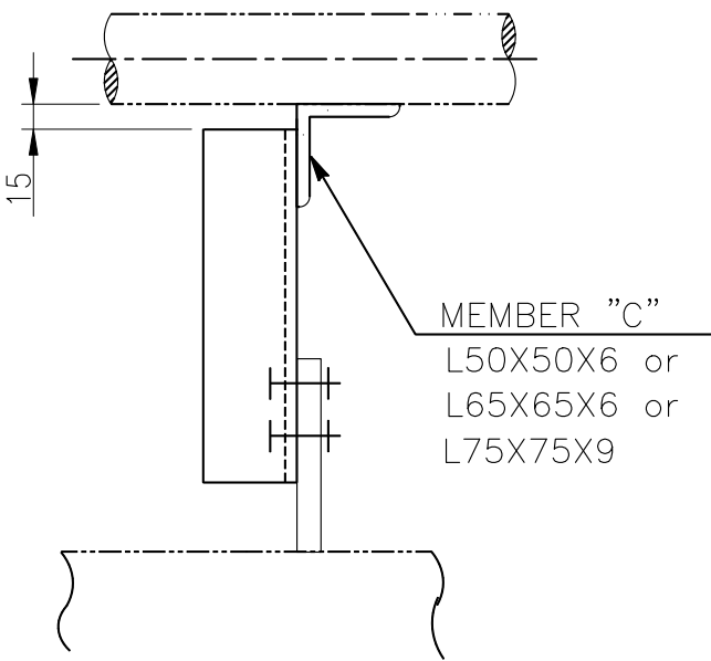
ELEV.
