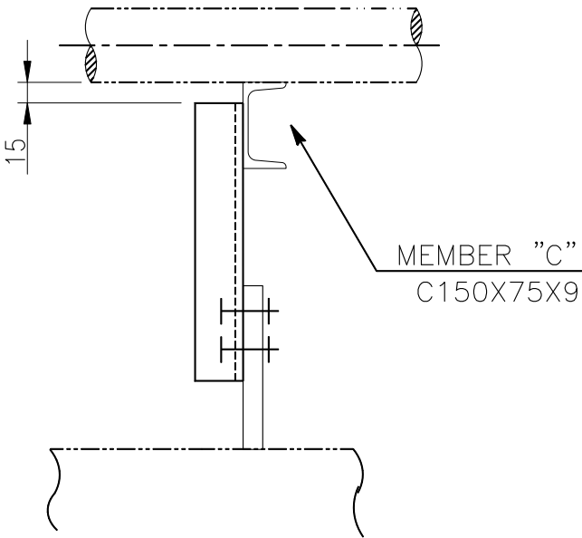
ELEV.
