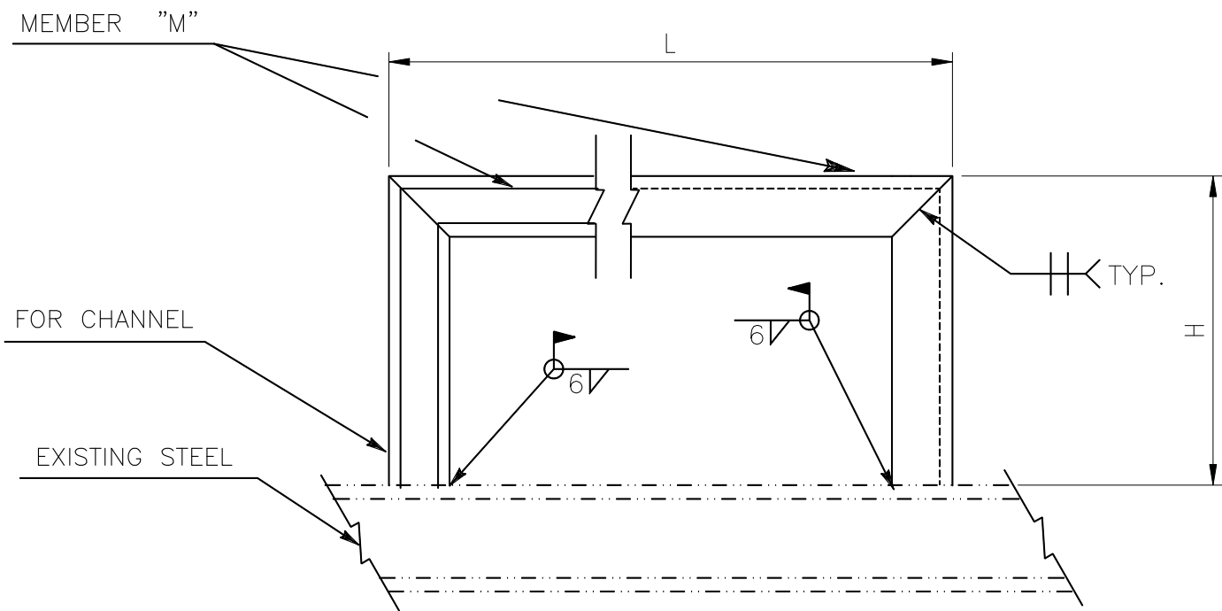
ELEV.
