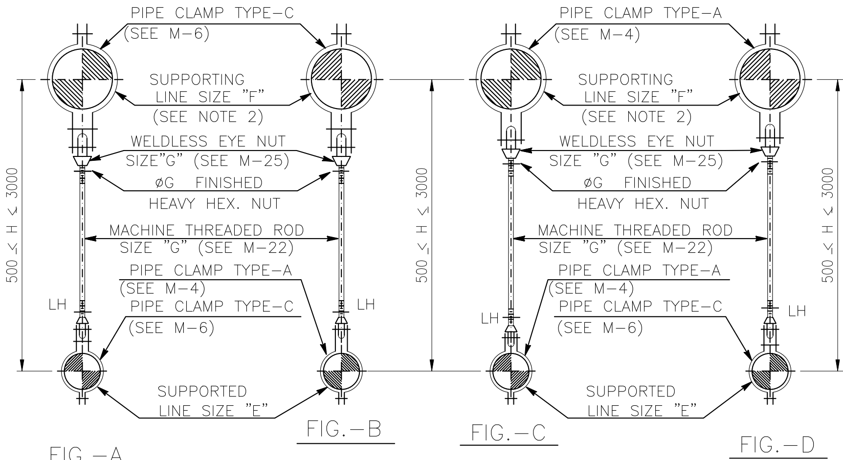
ELEV.
