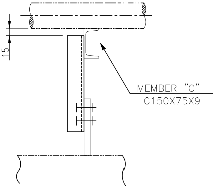
ELEV.
