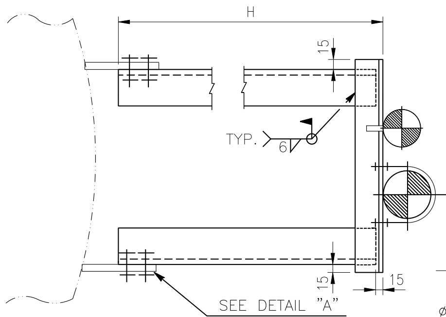
FIG. -C (PLAN VIEW)
