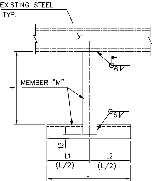
FIG.-B (ELEV.)
