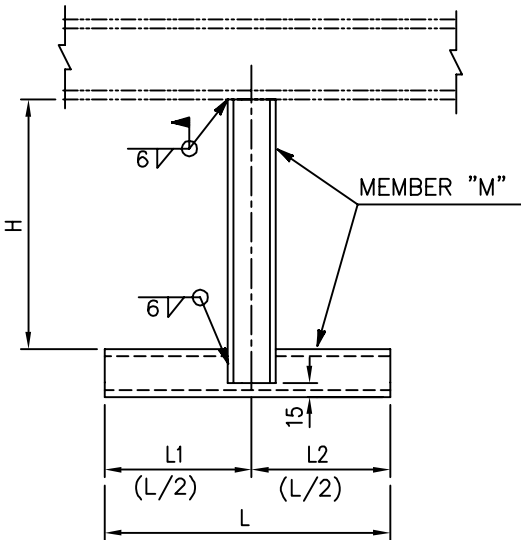
FIG.-B (ELEV.)
