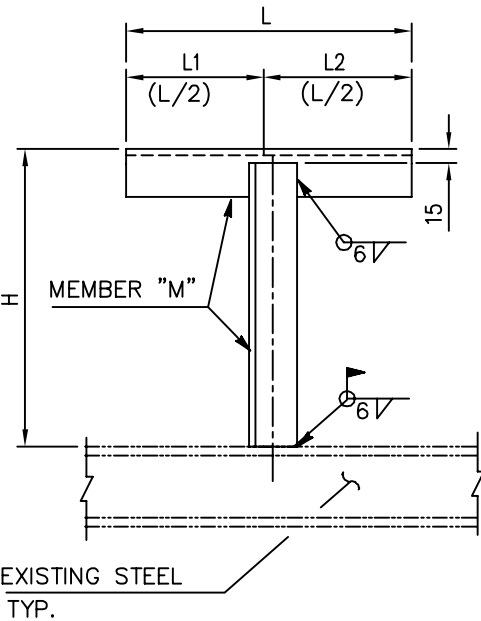
FIG.-A (ELEV.)
