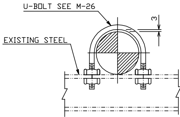
FIG.-A (SLIDE)
