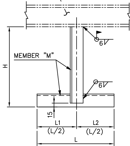
FIG.-B (ELEV.)
