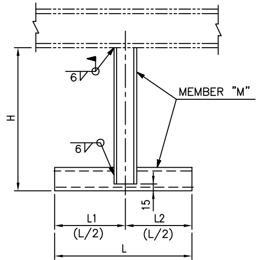
FIG.-B (ELEV.)
