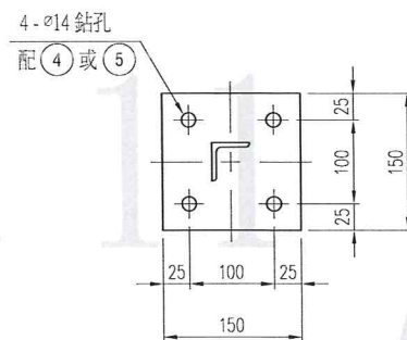
A-A 視圖
