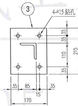
型式：SS13VB
