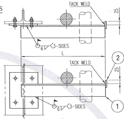
型式：SS13SB
