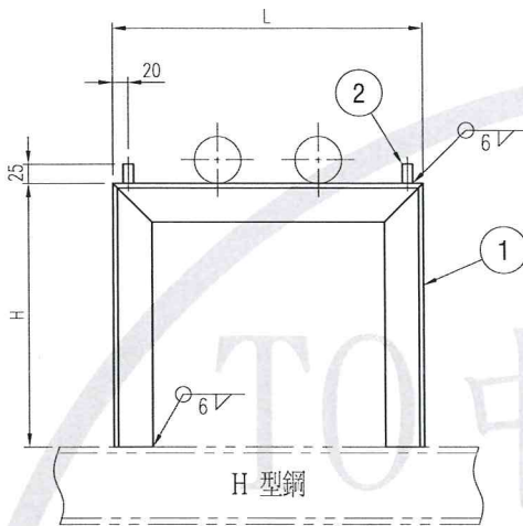
型式：SS5W
