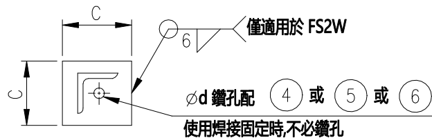
"E" - "E" 視圖
