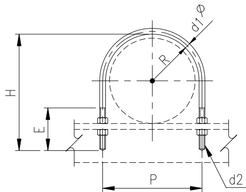
管線 4" (含) 以上安裝方式
