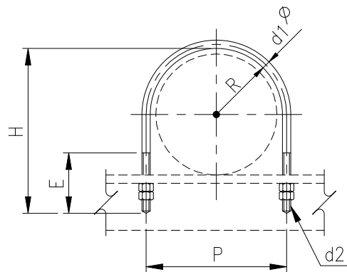
管線 4" 以下安裝方式
