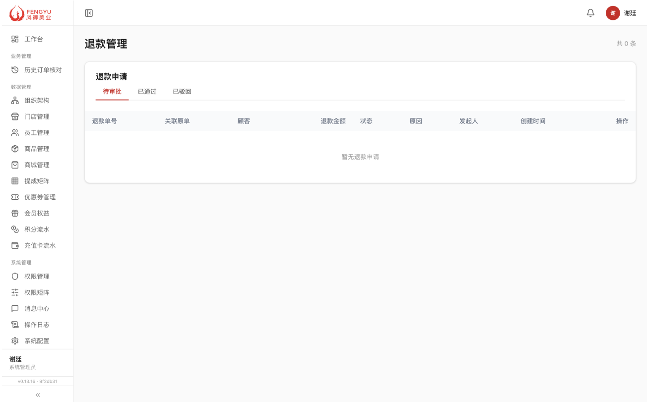
Figure 36: 退款页面
