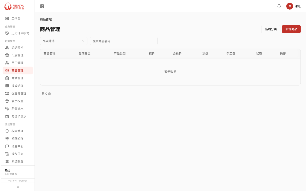
Figure 12: 商品列表页
