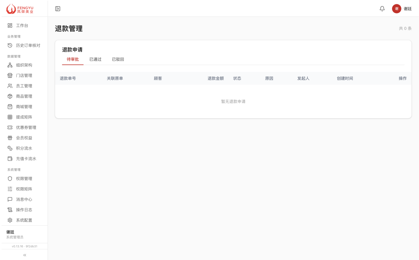
Figure 28: 退款页面
