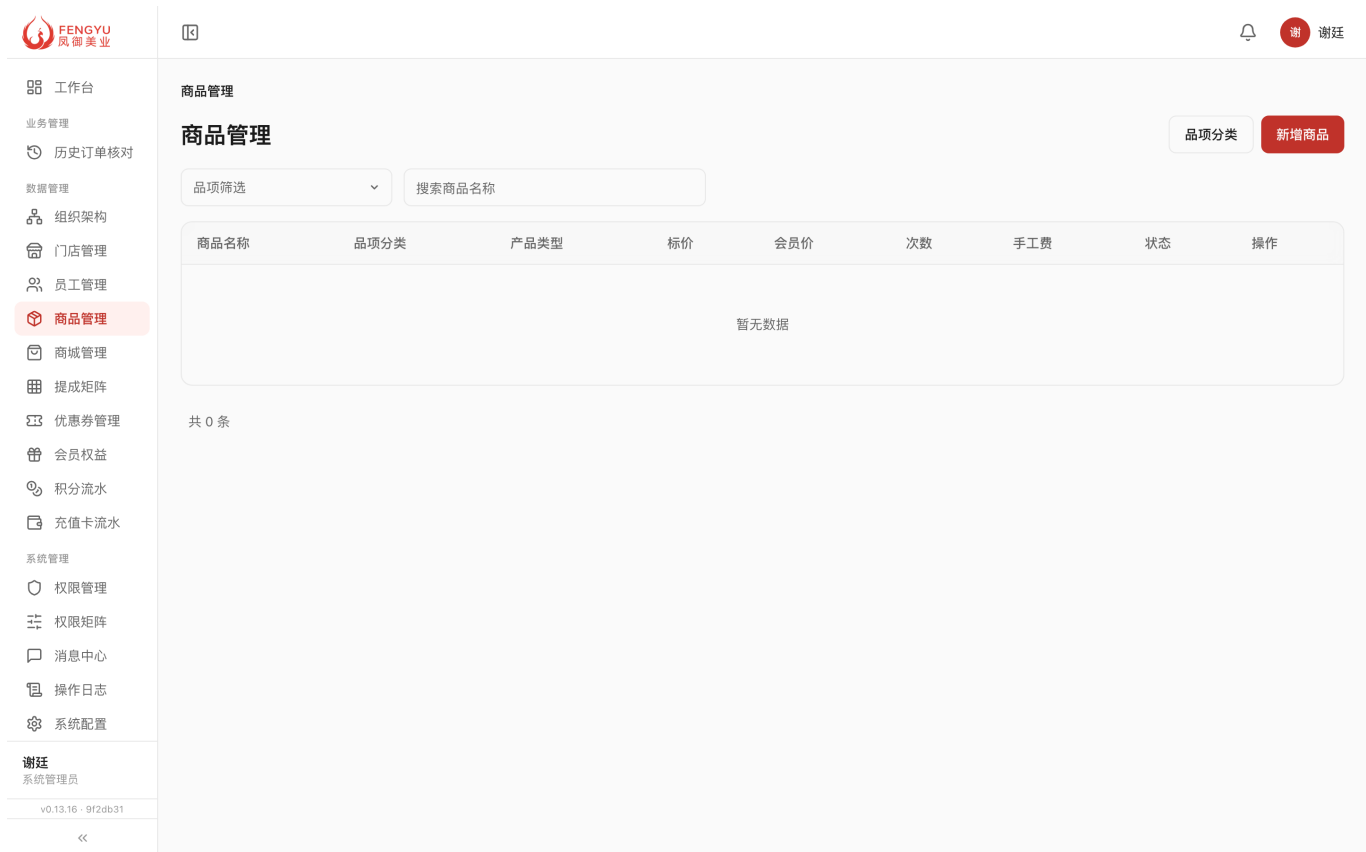
Figure 12: 商品列表页
