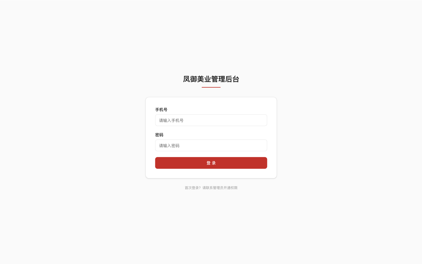
Figure 1: 登录页面
