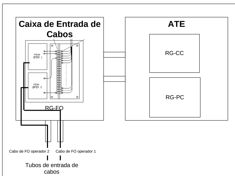
4.74 - Instalação do RG-FO em caixa de entrada de cabos
