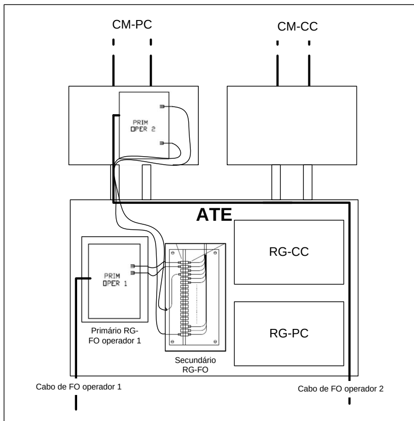
4.73 - Instalação do RG-FO no ATE inferior, desdobramento do primário de 2.º operador
