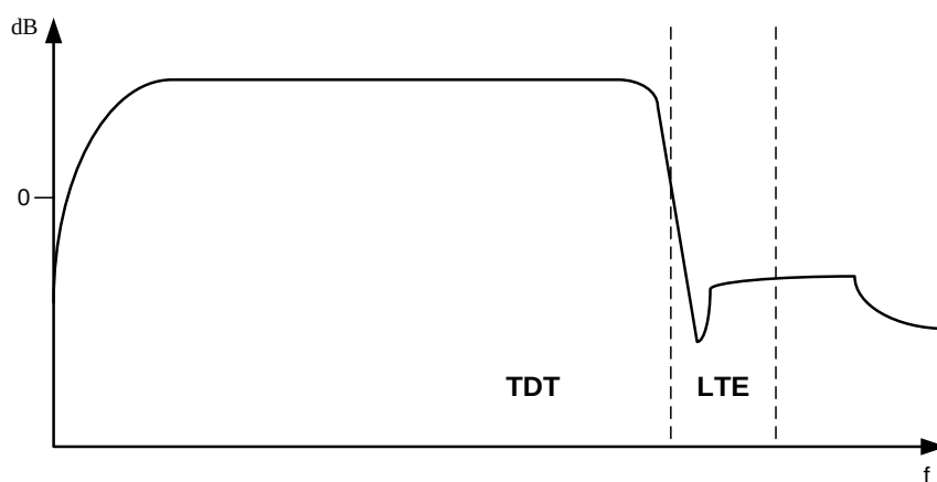
3.19 - Resposta de um amplificador com filtro integrado
