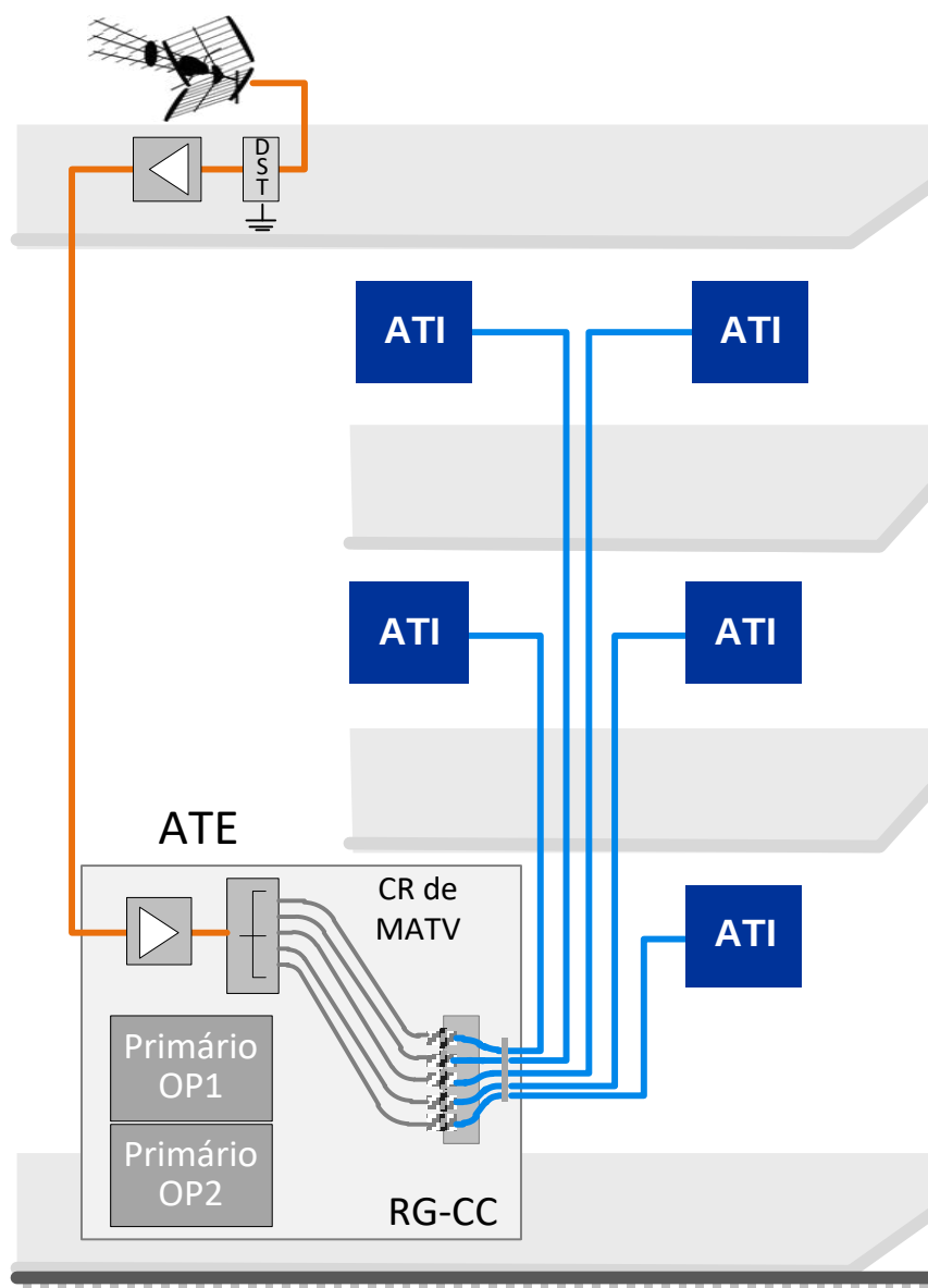
4.27 - Rede coletiva de cabos coaxiais - SCU
