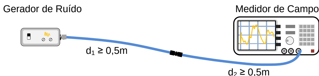
6.6 - Medida da referência
