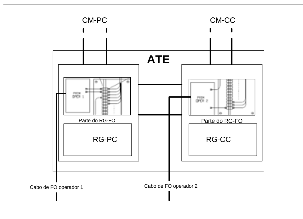
4.71 - Desdobramento do RG-FO nas caixas do ATE
