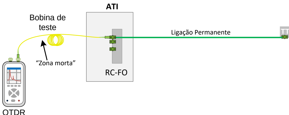
6.19 - Ensaio para determinação de falhas na ligação
