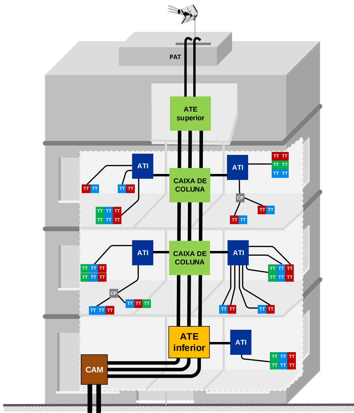
4.2 - Rede coletiva e individual de tubagens de um edifício ITED
