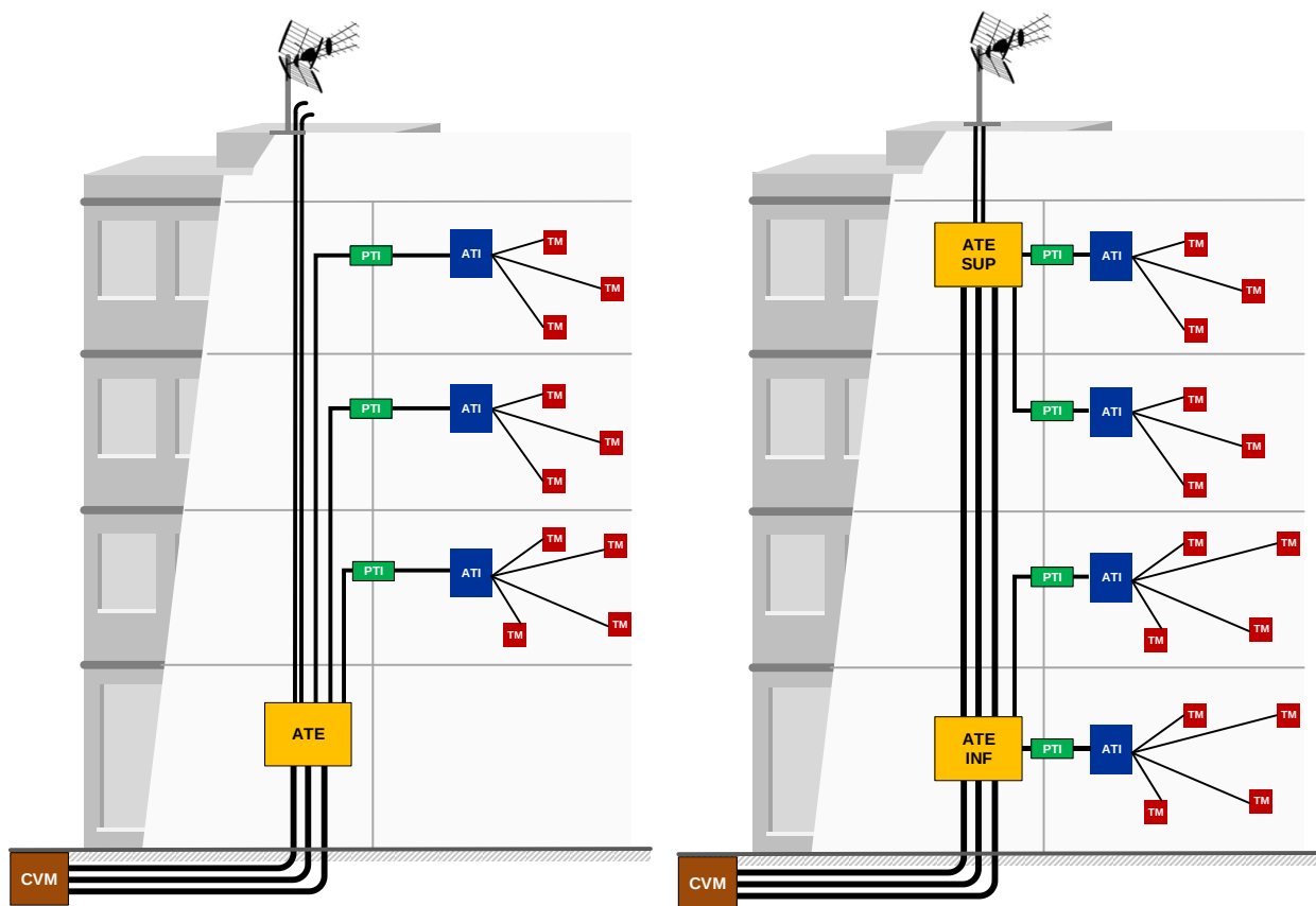
4.57 - Exemplos para a rede de tubagens – ITED4a
