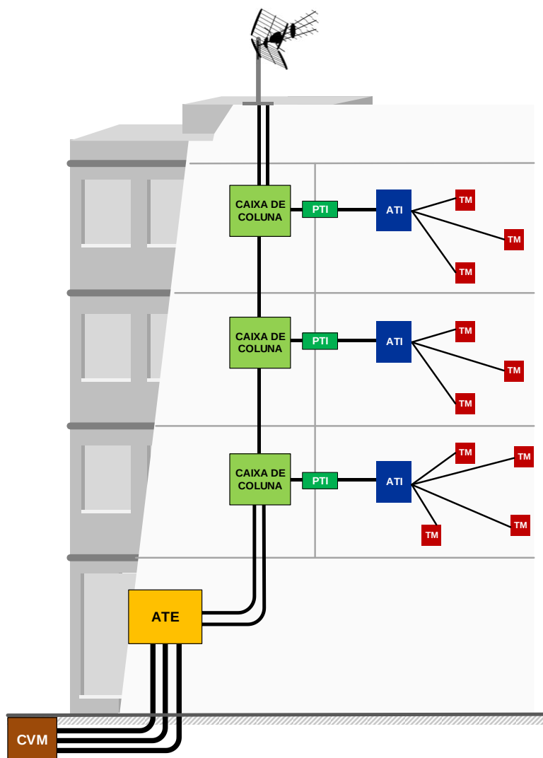
4.58 - Exemplo para a rede de tubagens – ITED4a
