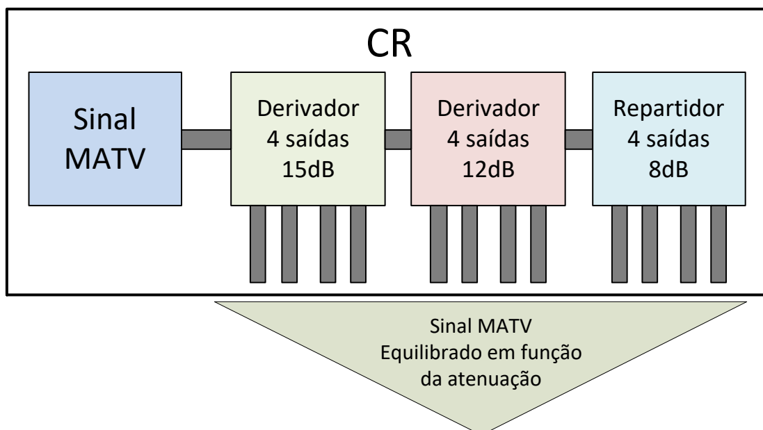
4.38 - Exemplo de dimensionamento da CR
