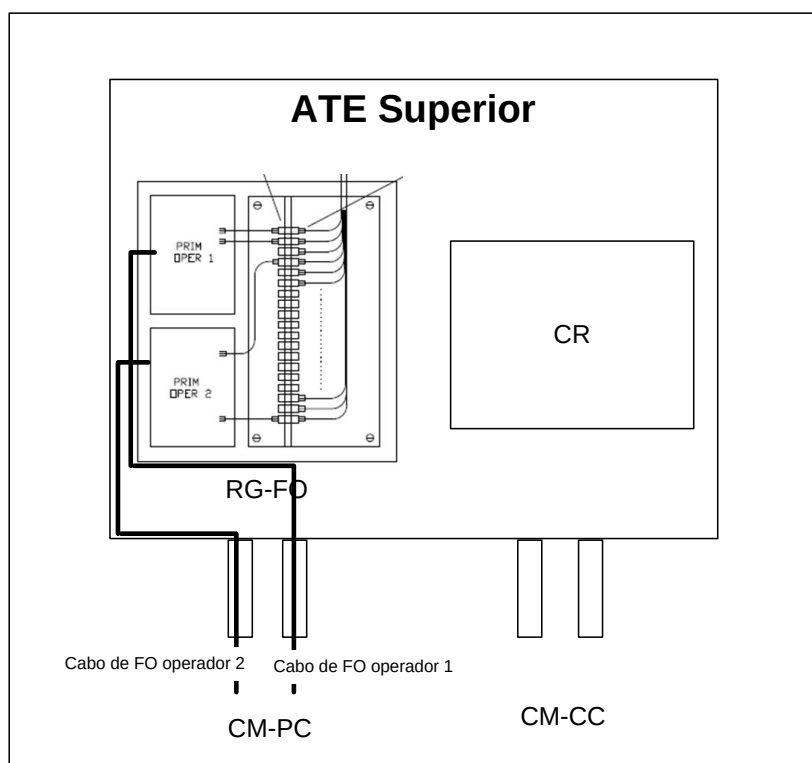
4.72 - Instalação do RG-FO no ATE superior
