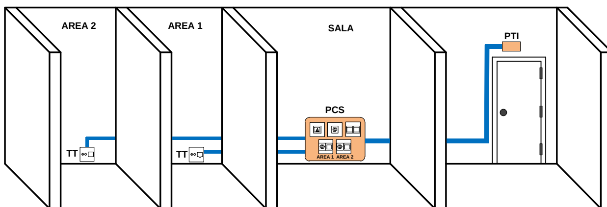
4.53- Exemplo de instalação de um PTI e de um PCS
