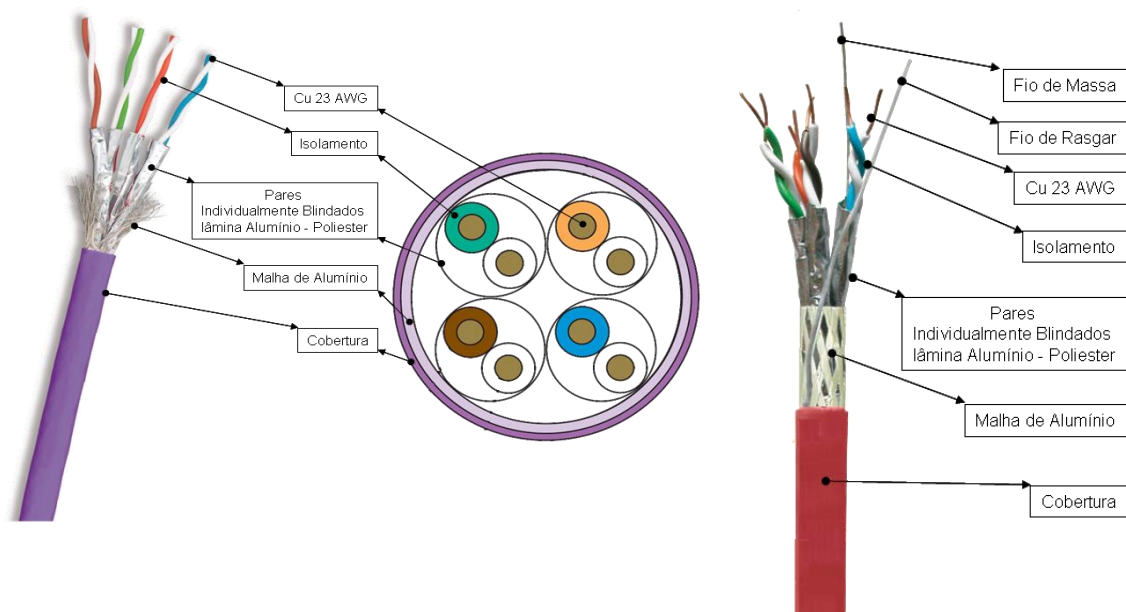
3.4 - Exemplo de cabo F/FTP, Cat. 7
