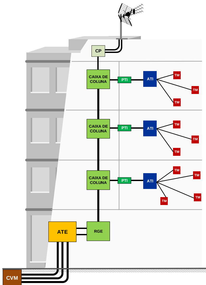
4.59 - Exemplo para a rede de tubagens
