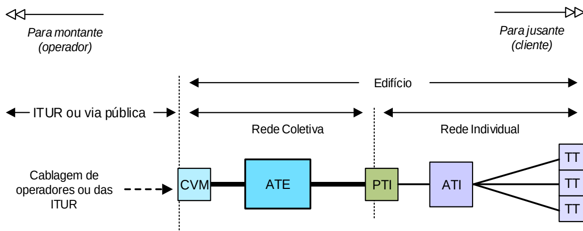
4.50 - Aplicação das ITED4a a um edifício residencial construído, com rede coletiva
