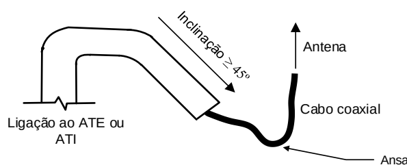
5.1 - Tubo da PAT
