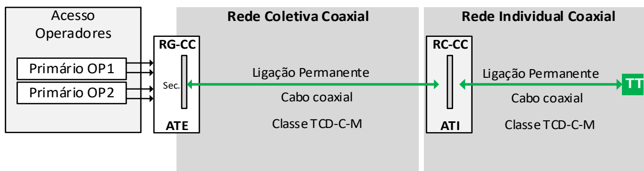
4.22 – Exemplo de uma rede coletiva e individual de cabo coaxial
