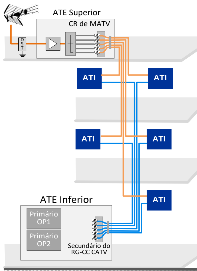
4.25 – Redes coletiva de cabos coaxiais – SCI
