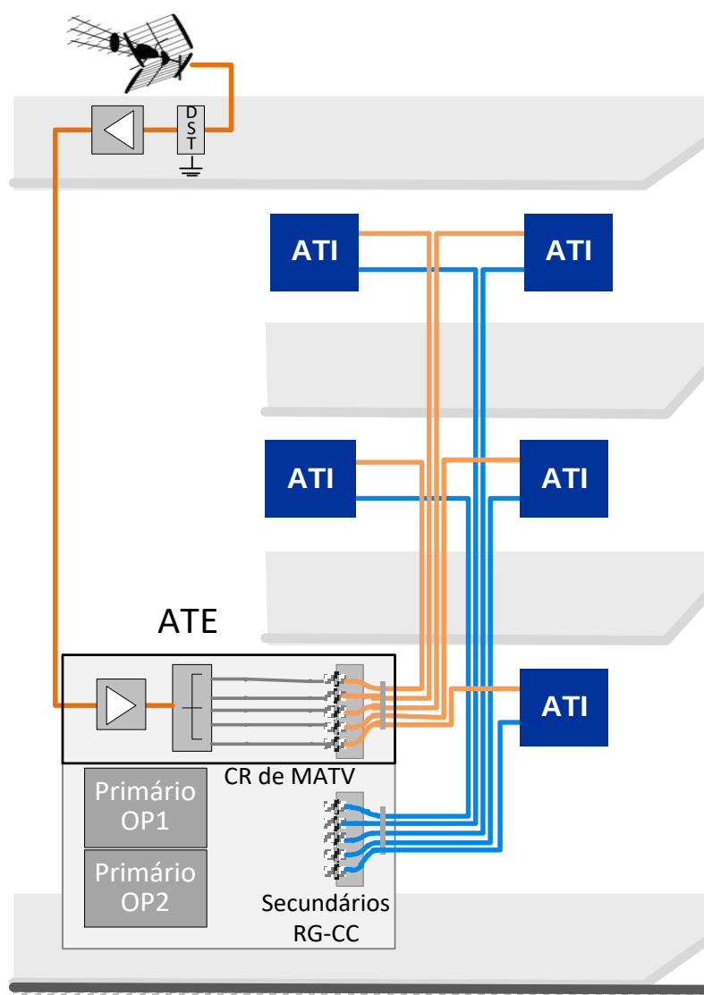
4.26 - Redes coletiva de cabos coaxiais – SCI
