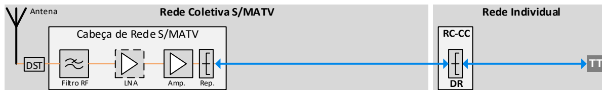
4.28 - Elementos constituintes de uma rede de S/MATV
