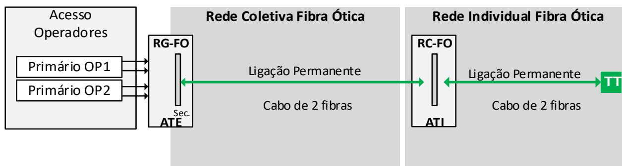
4.39 - Constituição de uma rede de FO
