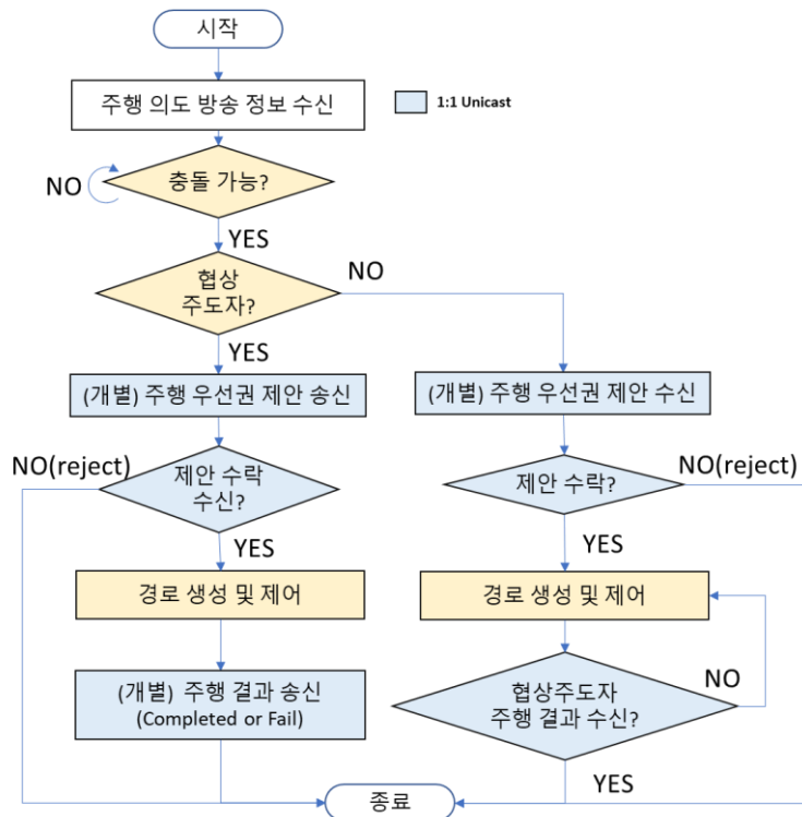
그림 8. Class C 주행협상전략 (1:1)
