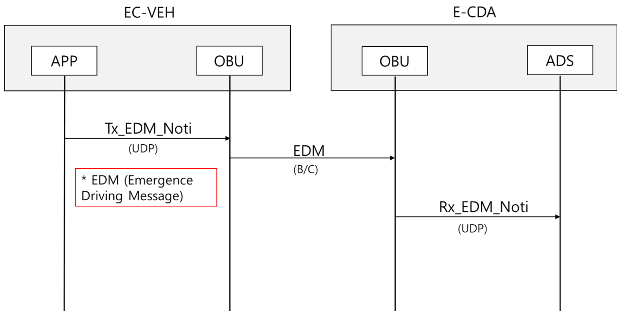
그림 11. E-CDA와 EC-VEH 간 긴급주행메시지(EDM) 공유를 통한 협력주행
