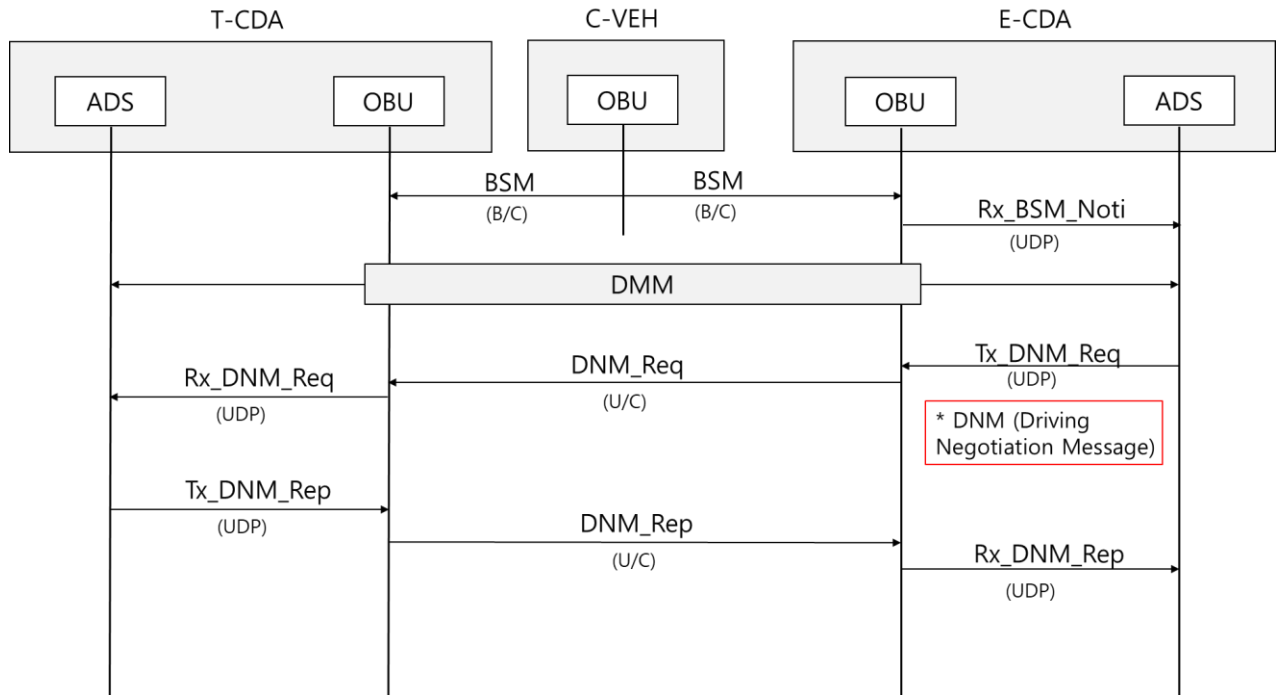
그림 9. E-CDA와 T-CDA 간 주행협상메시지(DNM)을 통한 협력주행 (* E-CDA가 협상 우선권을 가진 경우의 예시 임) // 주행결과 송.수신 추가 요청
