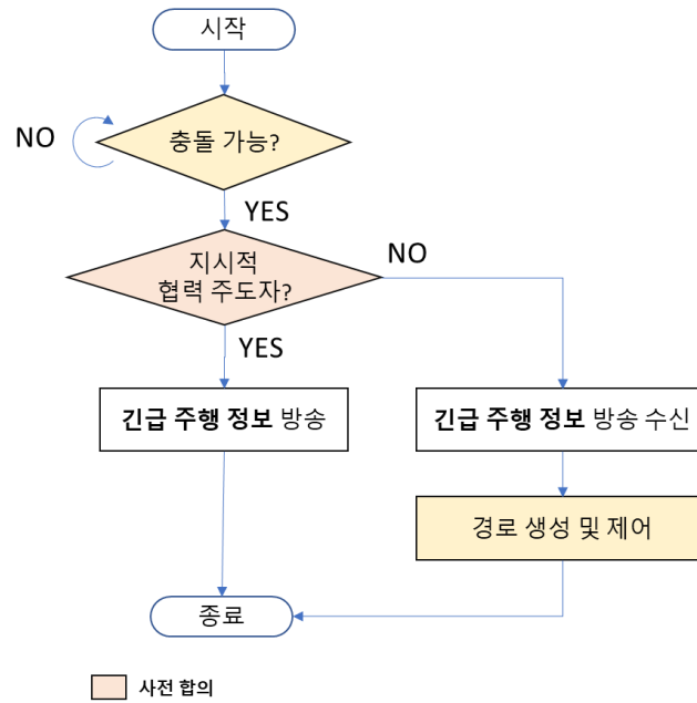
그림 10. Class D 주행협상전략
