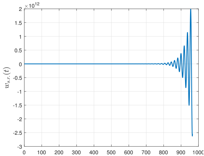
Рисунок 41: Переходная характеристика замкнутой системы при k = 0.1
