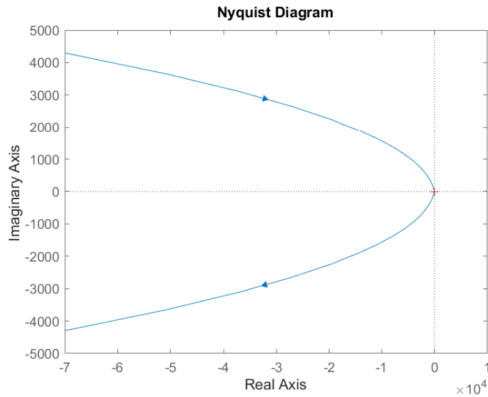
Рисунок 38: Годограф второй системы, k = 2
