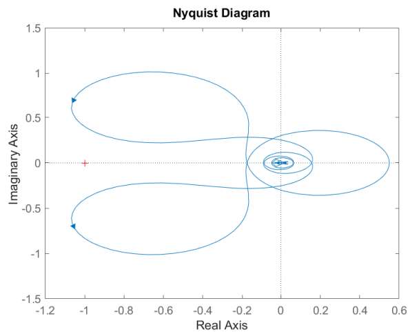
Рисунок 57: Годограф Найквиста второй системы при \tau = 0.7
