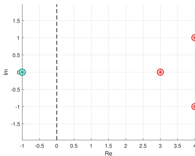
Рисунок 3: Карта нулей замкнутой системы
