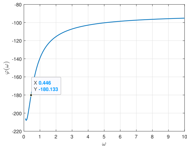
Рисунок 40: ФЧХ второй системы, k = 1
