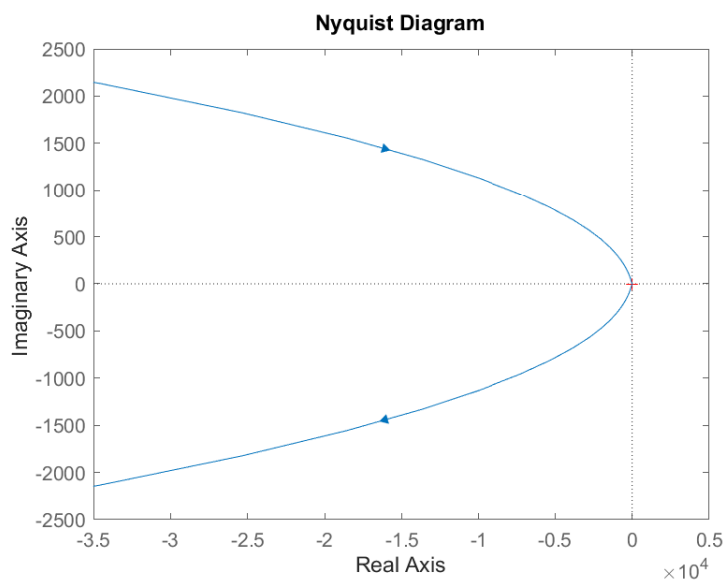
Рисунок 35: Годограф второй системы, k = 1
