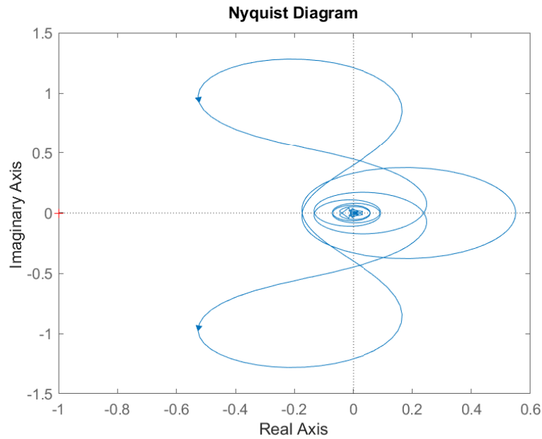
Рисунок 58: Годограф Найквиста второй системы при \tau = 1
