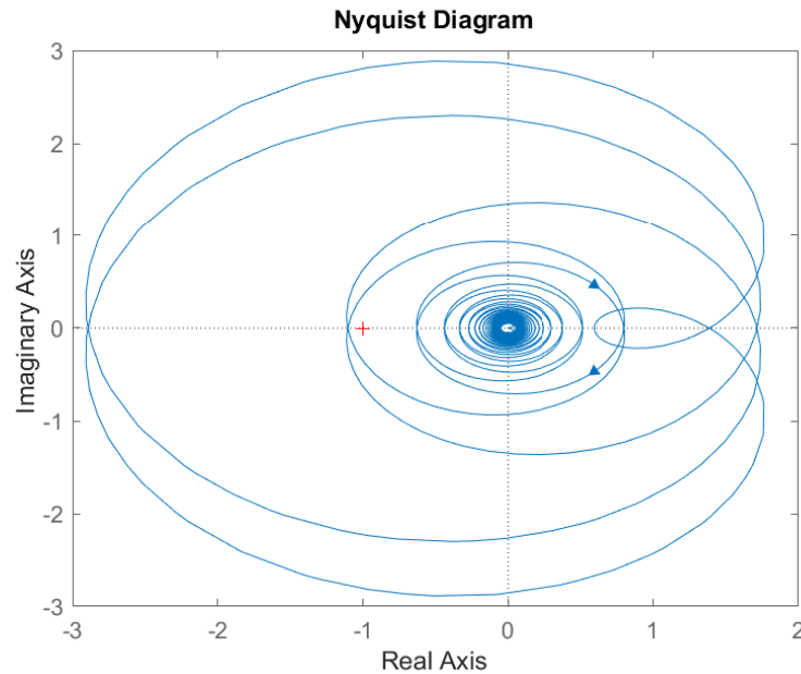
Рисунок 48: Годограф Найквиста первой системы при \tau = 1
