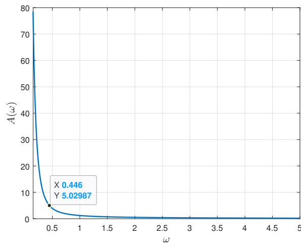
Рисунок 39: АЧХ второй системы, k = 1
