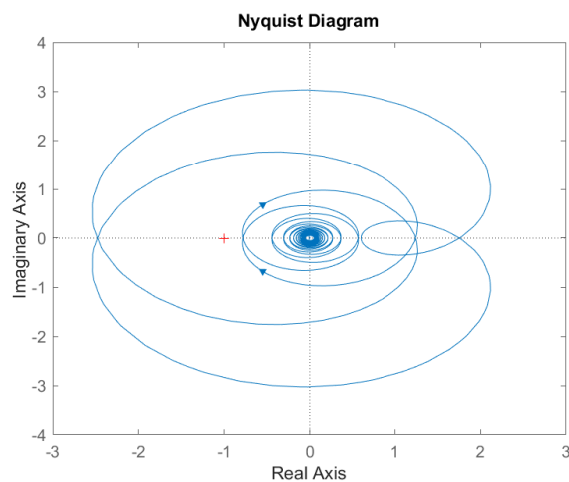
Рисунок 47: Годограф Найквиста первой системы при \tau = 0.7
