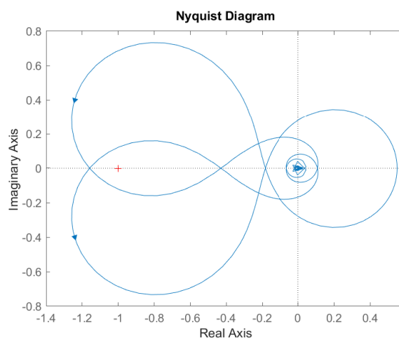
Рисунок 55: Годограф Найквиста второй системы при \tau = 0.5
