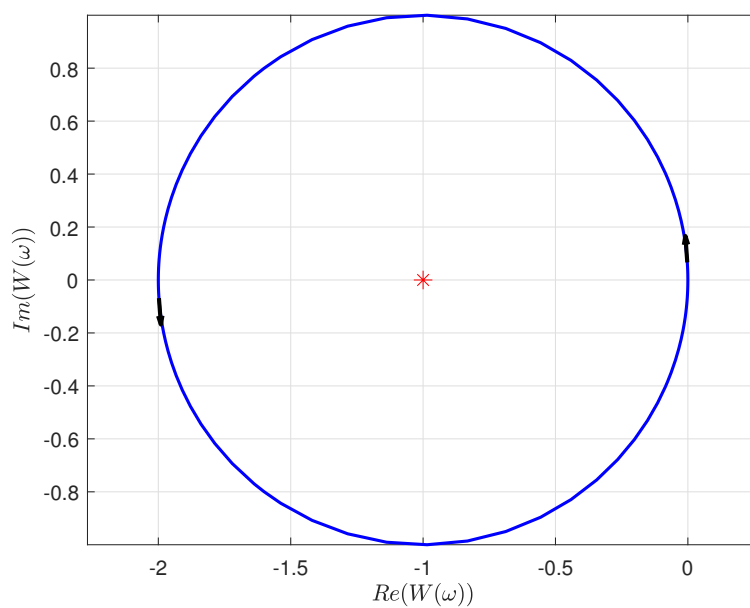
Рисунок 7: Годограф Найквиста
