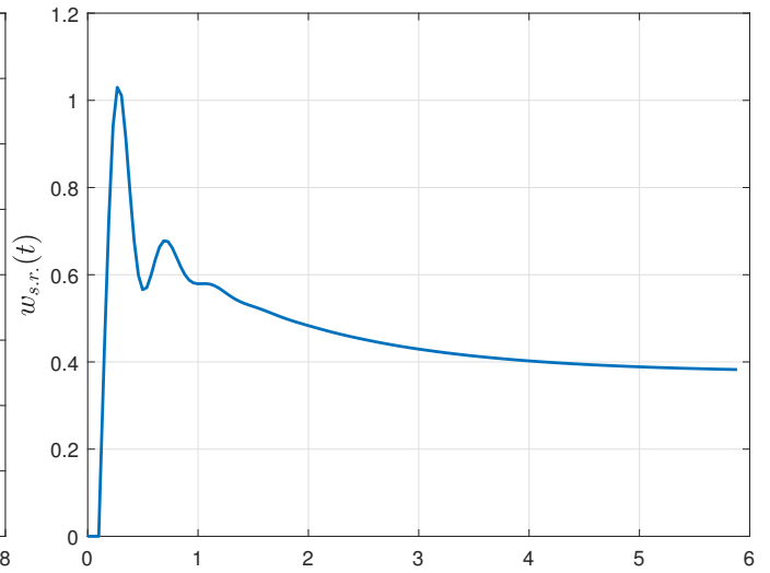
Рисунок 51: Переходная характеристика первой системы при \tau = 0.1
