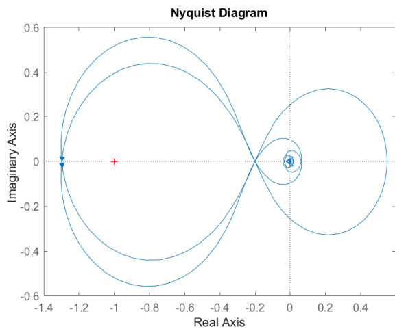
Рисунок 56: Годограф Найквиста второй системы при \tau = 0.3
