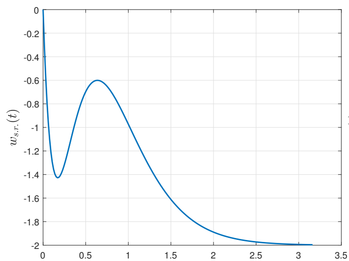
Рисунок 14: Переходная характеристика разомкнутой системы
