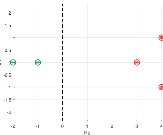
Рисунок 4: Карта полюсов замкнутой системы
