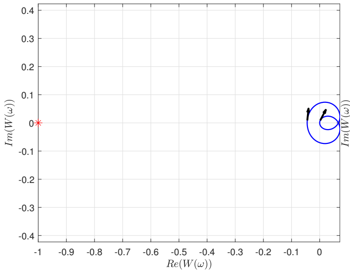
Рисунок 29: Годограф первой системы, k = 1/5
