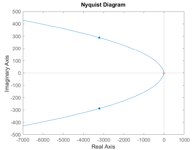
Рисунок 37: Годограф второй системы, k = 0.2
