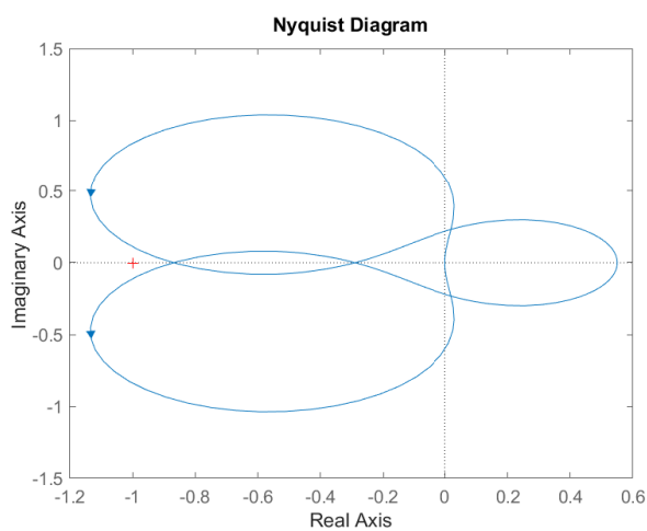
Рисунок 54: Годограф Найквиста второй системы при \tau = 0
