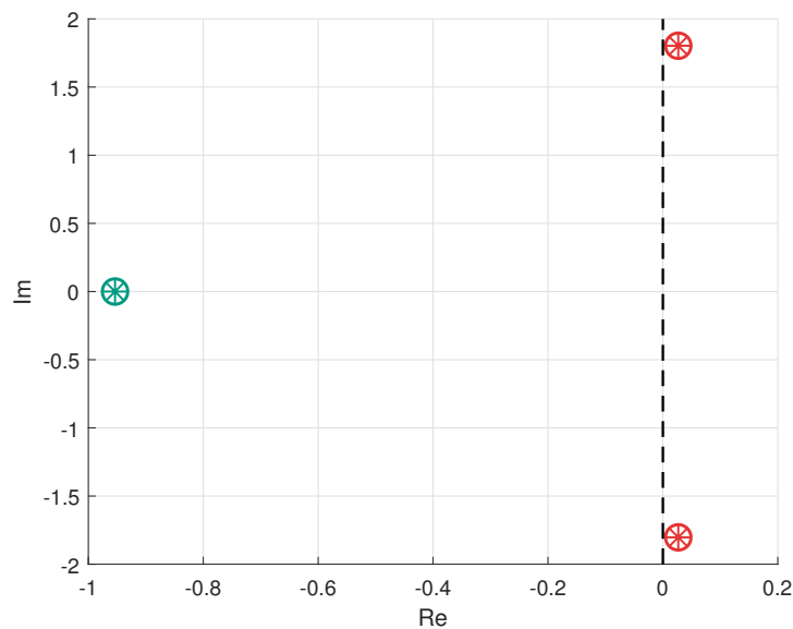
Рисунок 59: Карта полюсов разомкнутой системы при отсутствии запаздывания
