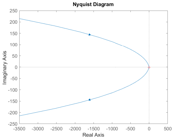
Рисунок 36: Годограф второй системы, k = 0.1
