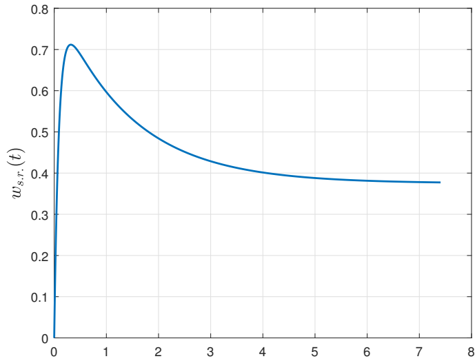
Рисунок 50: Переходная характеристика первой системы при \tau = 0
