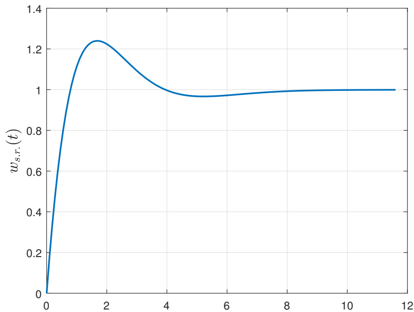
Рисунок 43: Переходная характеристика замкнутой системы при k = 2
