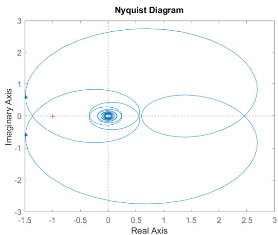
Рисунок 46: Годограф Найквиста первой системы при \tau = 0.3
