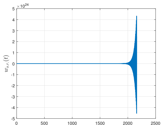
Рисунок 61: Переходная характеристика второй системы при \tau = 0
