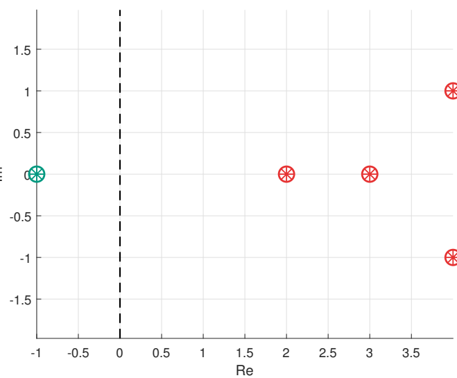
Рисунок 2: Карта полюсов разомкнутой системы
