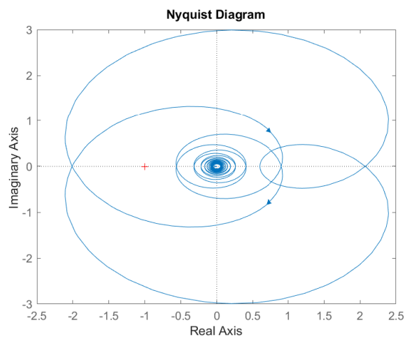
Рисунок 45: Годограф Найквиста первой системы при \tau = 0.5
