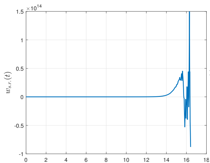
Рисунок 5: Переходная характеристика разомкнутой системы
