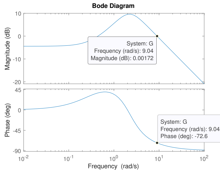
Рисунок 49: Графики ЛАЧХ и ЛФЧХ первой системы при \tau = 0
