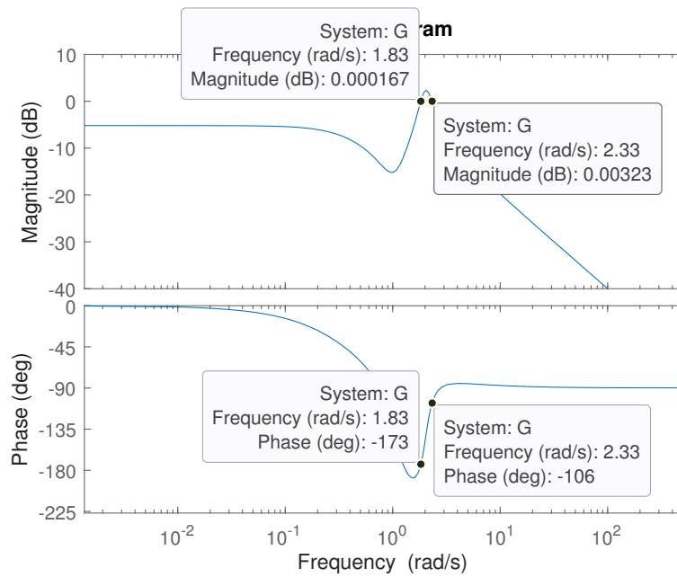
Рисунок 60: Графики ЛАЧХ и ЛФЧХ второй системы при \tau = 0
