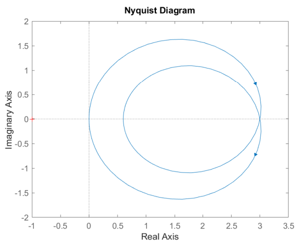
Рисунок 44: Годограф Найквиста первой системы при \tau = 0
