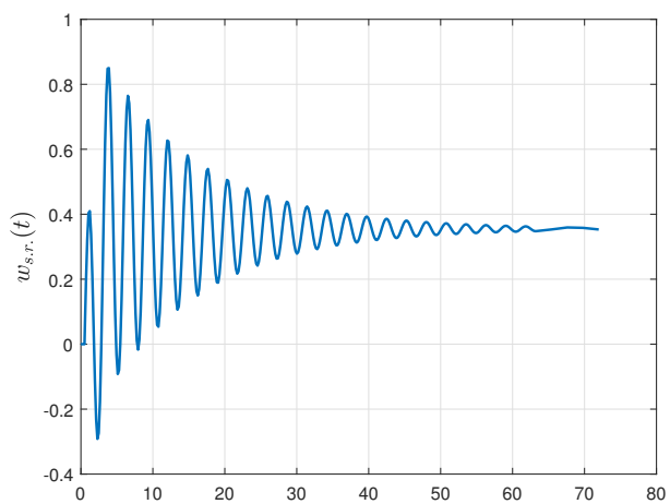
Рисунок 63: Переходная характеристика второй системы при \tau = 0.5
