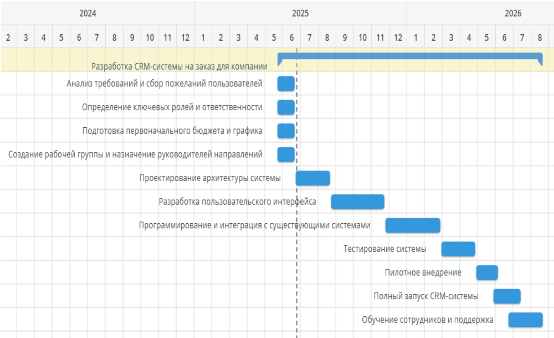
ДИАГРАММА ГАНТА
